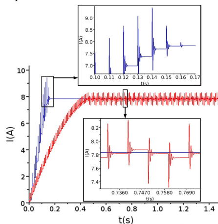
Figura 14: Variación de la corriente en el inductor en función del tiempo.
