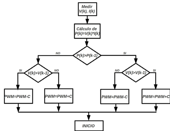
Figura 8: Diagrama de flujo del algoritmo P&O.
