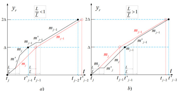
Figura 8: Influencia de los errores de modelado en el parámetro L . a) Respuesta de la realimentación para L/\bar{L} < 1 . b) Respuesta de la realimentación para L/\bar{L} > 1 .
