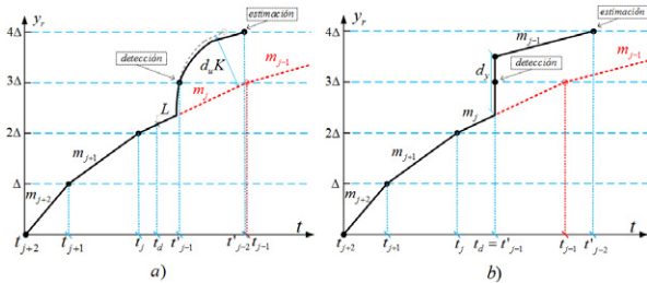
Figura 7: Fases de detección y estimación en condiciones de perturbación. a) Respuesta de la realimentación ante una perturbación a la entrada. b) Respuesta de la realimentación ante una perturbación a la salida. Las líneas rayadas rojas denotan el comportamiento ideal sin perturbación. Las líneas continuas negras denotan el comportamiento en condiciones de perturbación escalón.
