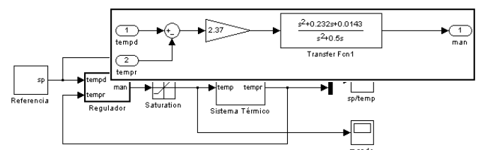
Figura 10. Cambio del controlador diseñado por el usuario.
