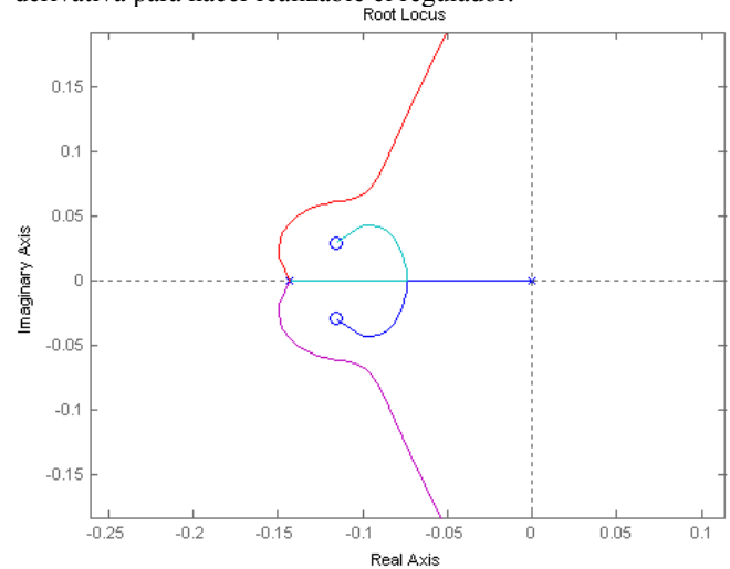
Figura 9. Lugar de las raíces del sistema térmico con red de compensación.
