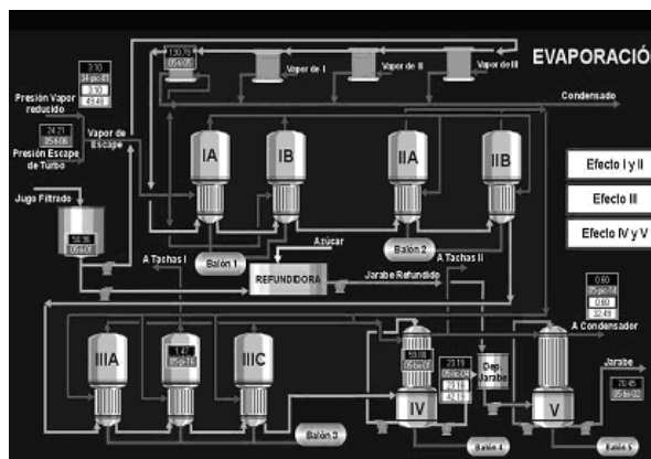
Figura 4. Pantalla original del área Evaporación del simulador del CTA.
