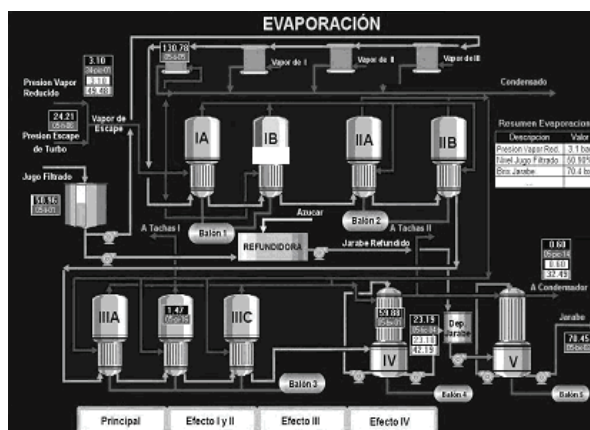
Figura 5. Pantalla modificada del área Evaporación del simulador del CTA atendiendo a los comentarios de mejoras expuestos en la sección 4.
