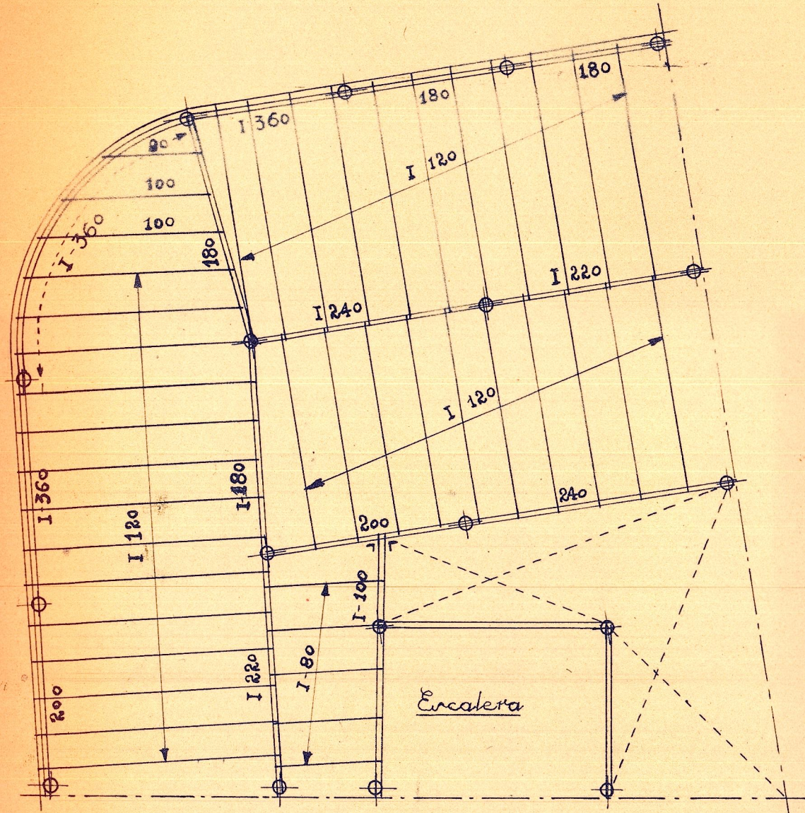
2ª Planta
