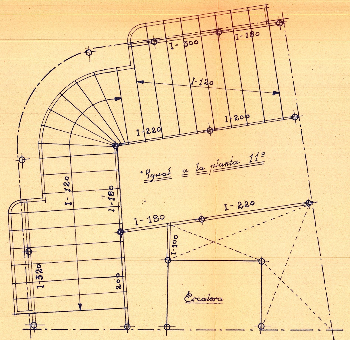
Planta 12ª
