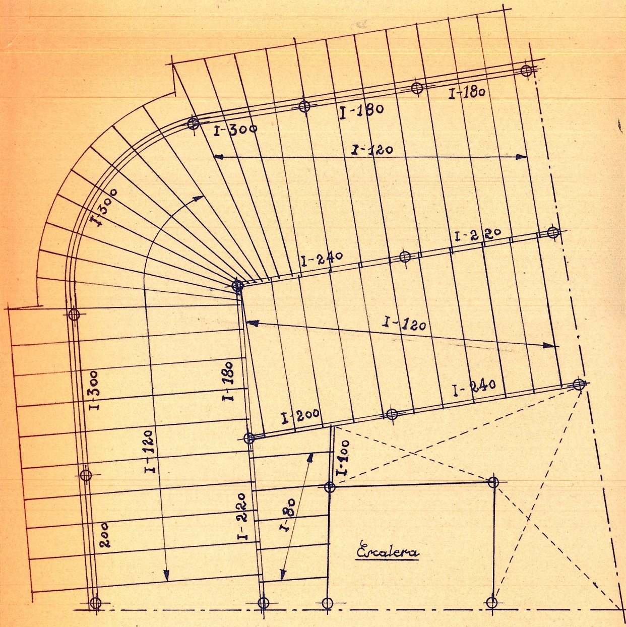
Planta 11ª
