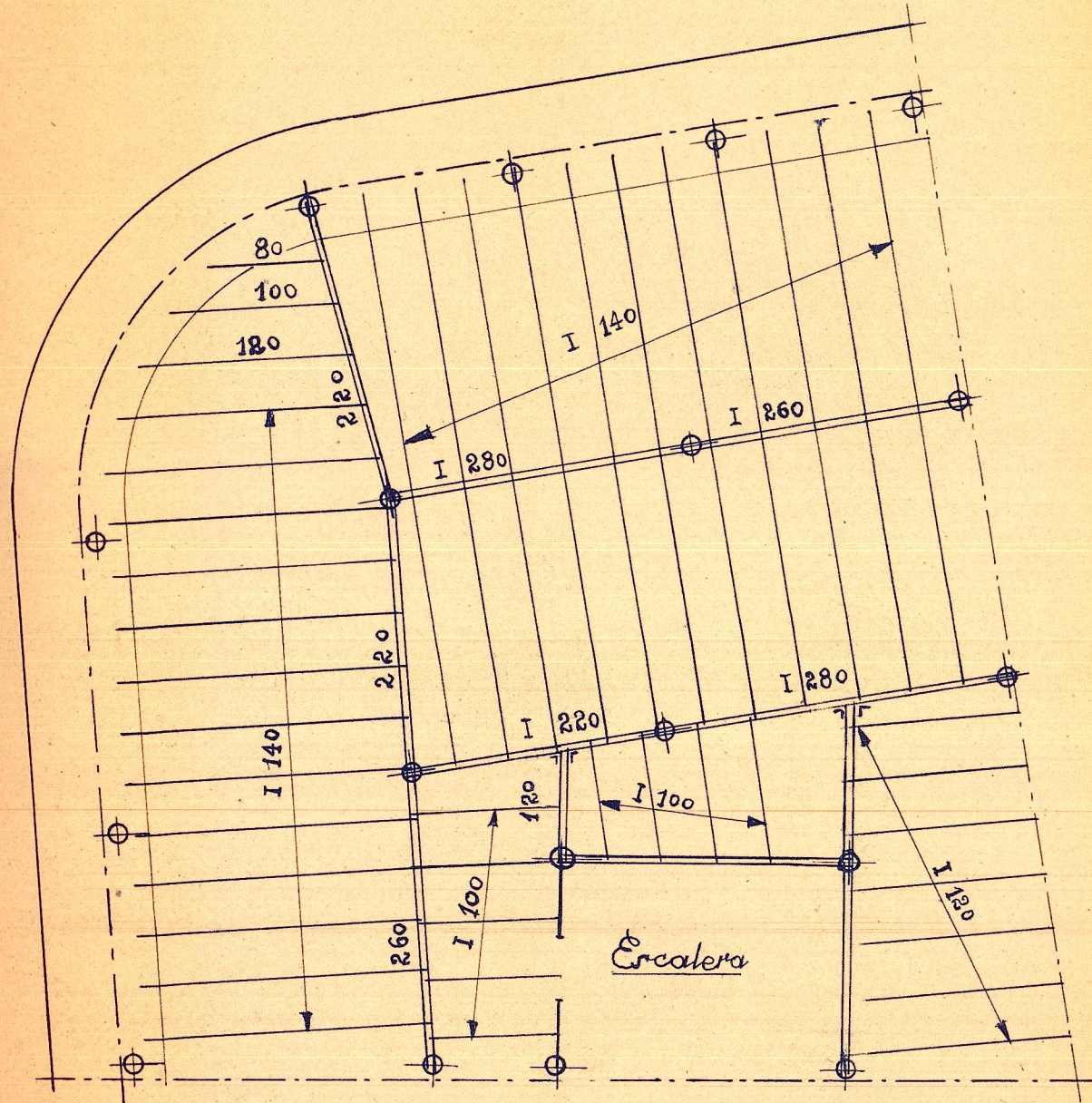
1ª Planta
