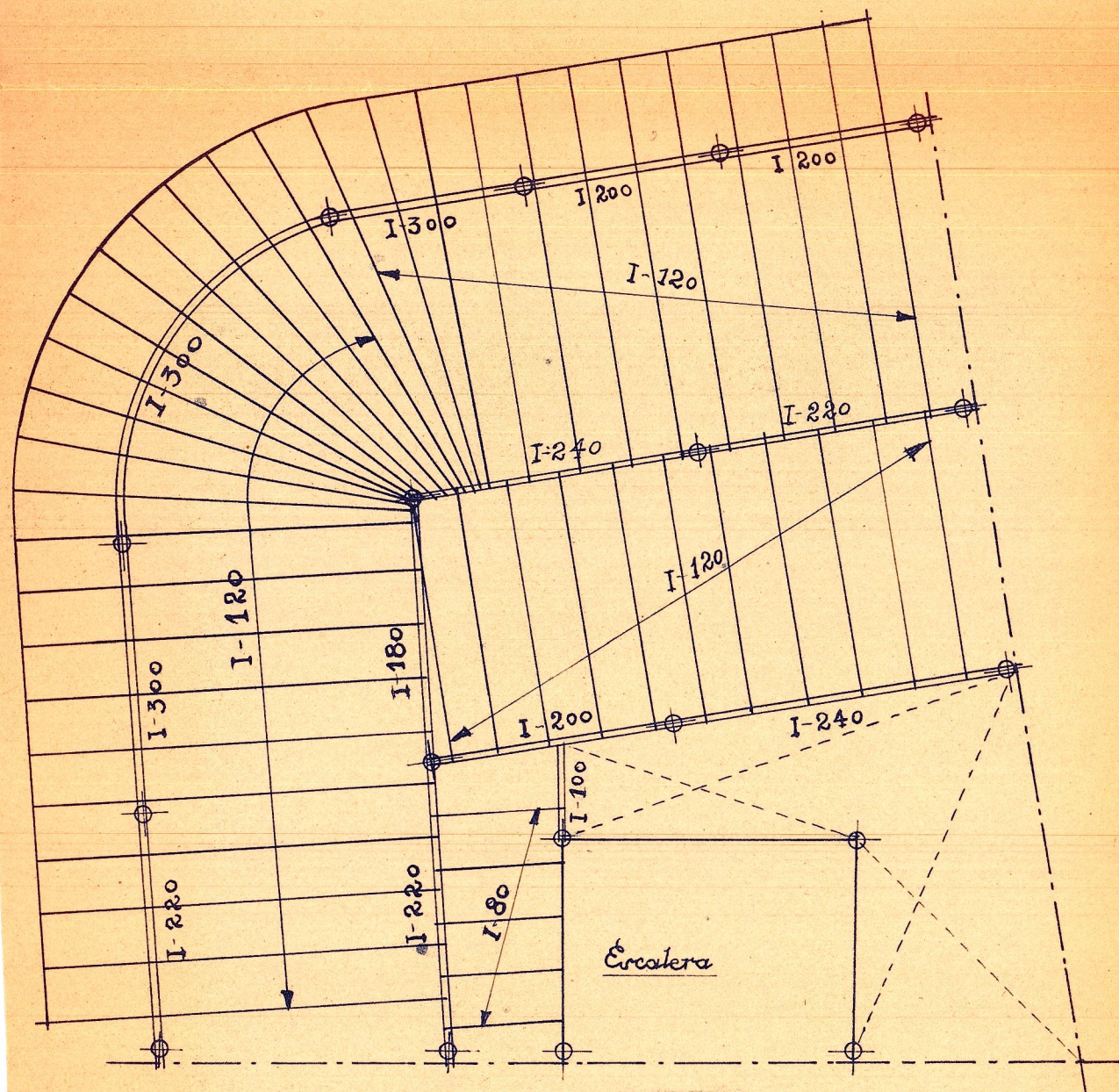
Planta 10ª
