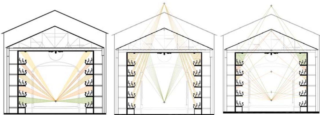
Figura 6. Sección longitudinal central del Teatro Principal. Llegada del sonido directo a todas las localidades
