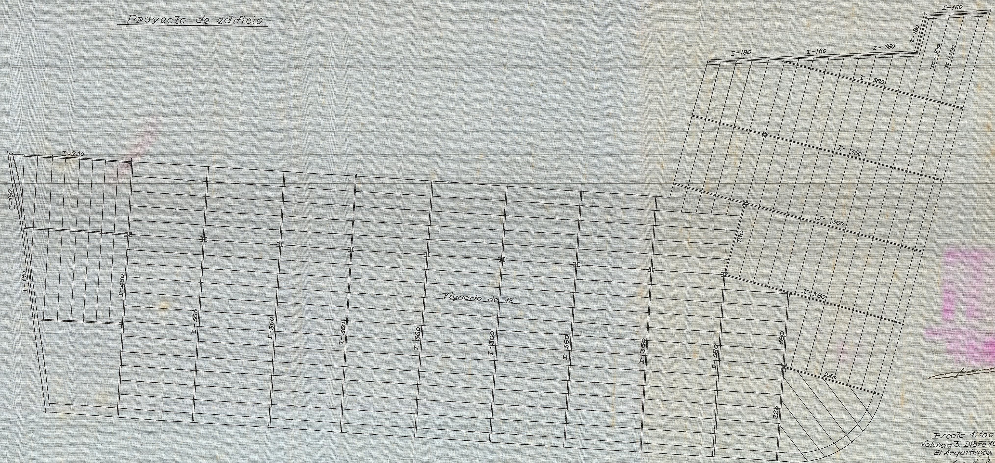
Planta de entramados 2ª a 5ª
