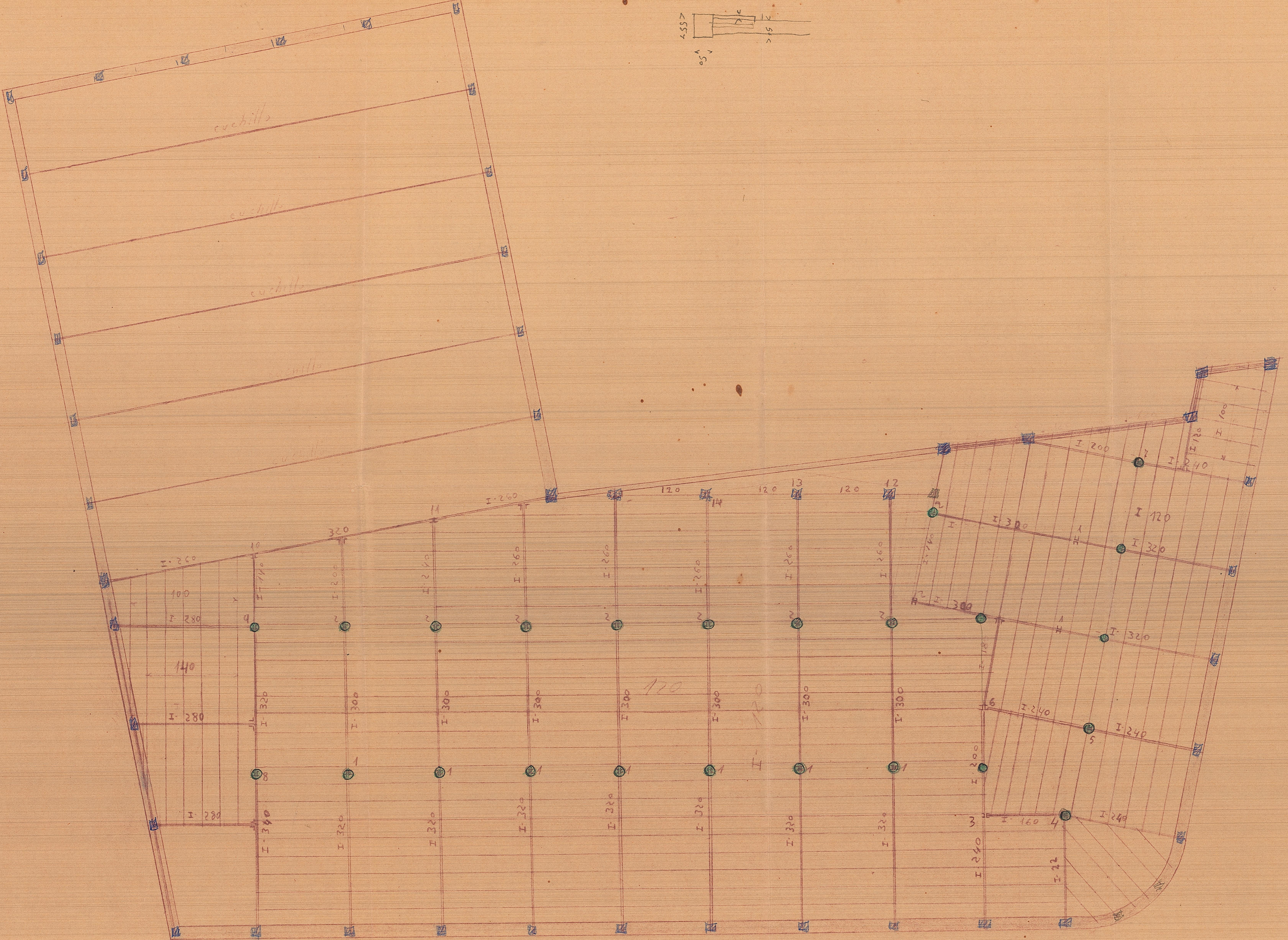
PLANTA 1ª
