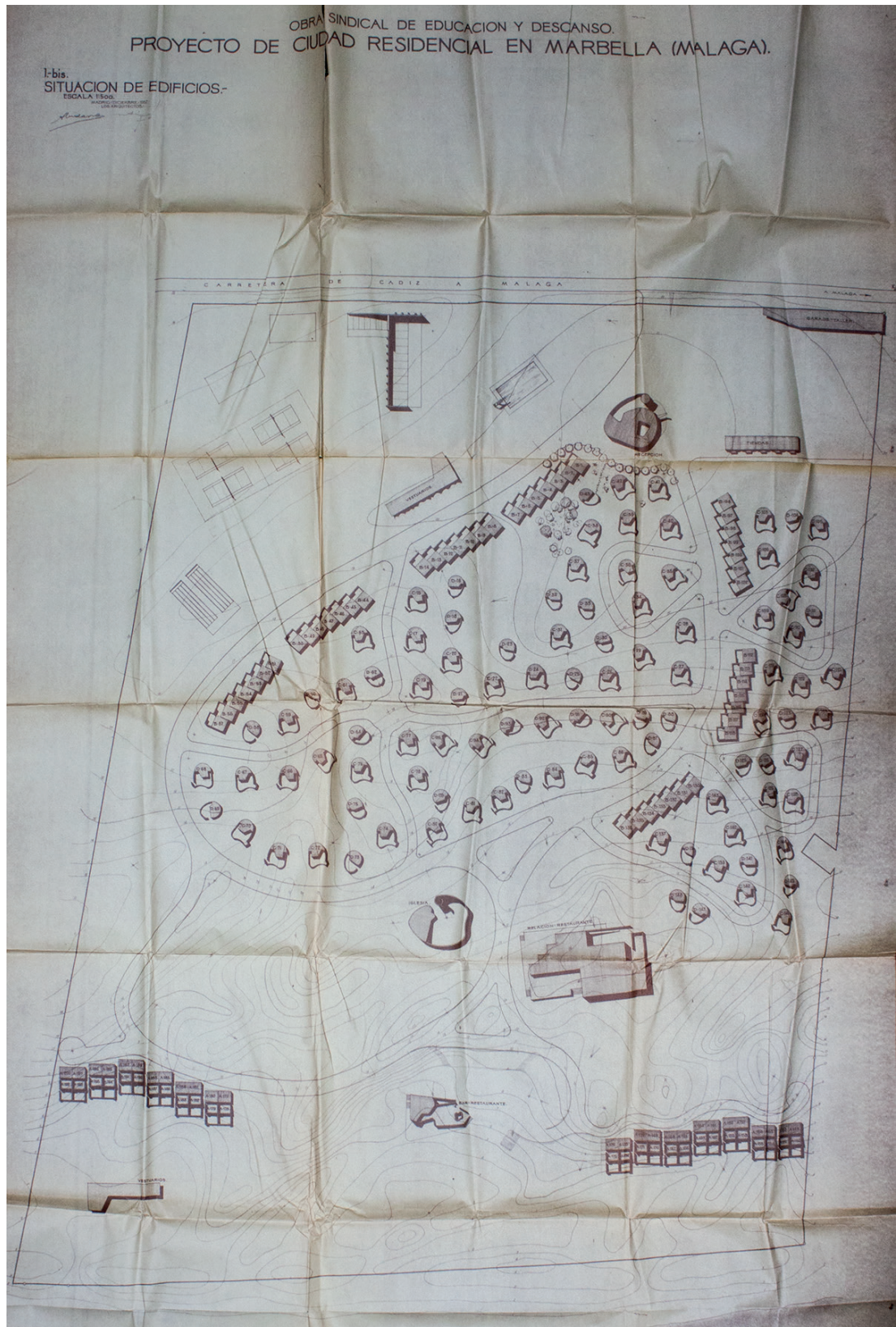
Figura 5. Ciudad Residencial en Marbella. Plano General (1957).
