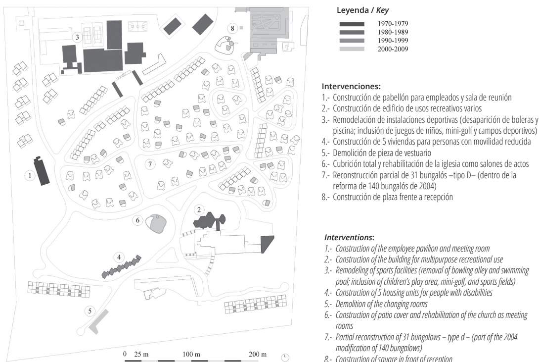
Figura 10. Planimetría actualizada de la Residencia de Tiempo Libre de Marbella con datación de las intervenciones de nuevas construcciones, ampliaciones y demoliciones (2018).
