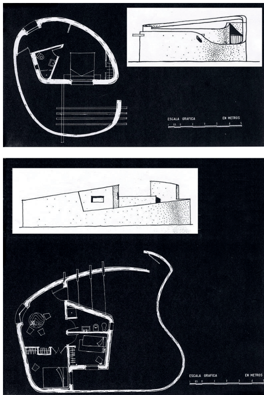
Figura 6. Arriba Izquierda: "Alzado y planta del hotel Tipo A". Proyecto original (1956). Abajo Izquierda: "Planta y alzado del hotel Tipo B". Proyecto original (1956). Derecha: "Planta del hotel Tipo C". Proyecto original (1956).
