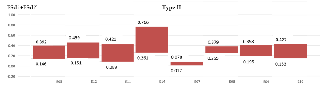
Figure 13. Area delamination factor range Type II (FS di + FS di ' ).
