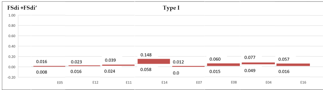
Figure 12. Area delamination factor range Type I (FS di + FS di ' ).
