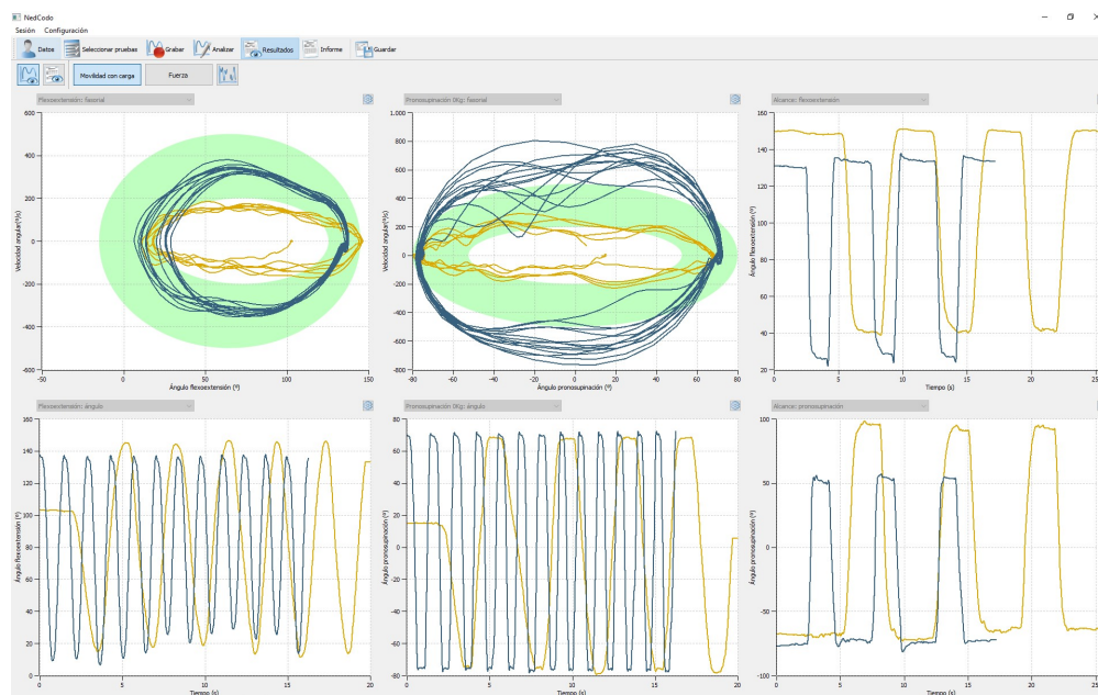
Figura 2: Ejemplo de pantalla de resultados de una valoración funcional de codo mediante el sistema NedCodo/IBV. Resultados de las pruebas de movilidad con carga.
