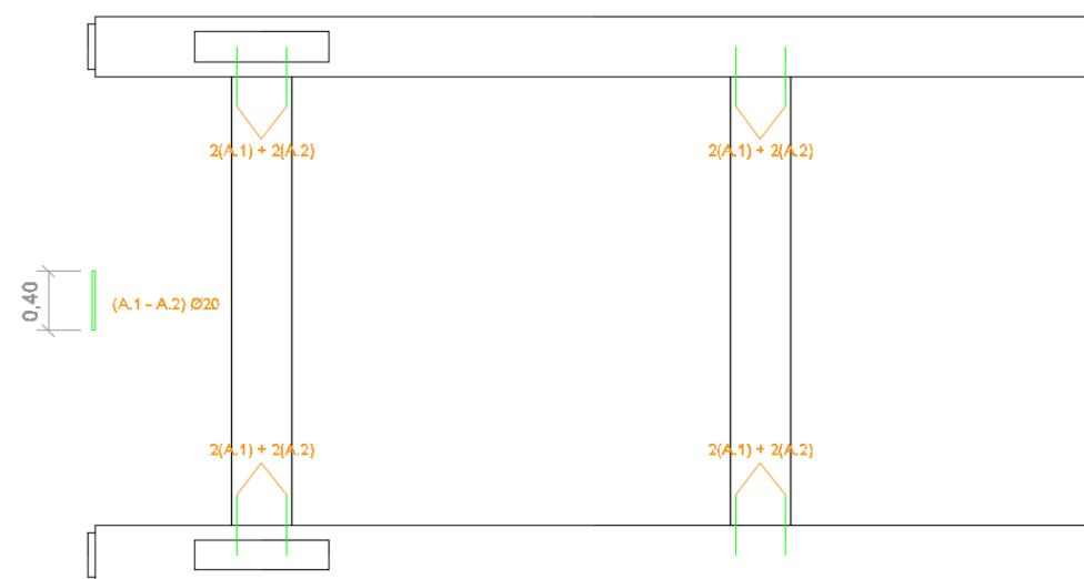
Figura 56 Detalle unión viga transversal – viga longitudinal
