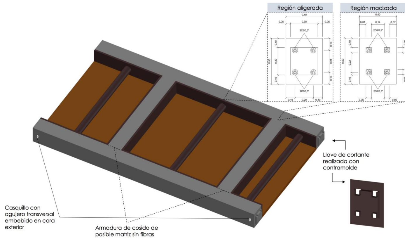
Figura 63 Módulo de tablero hormigonado
