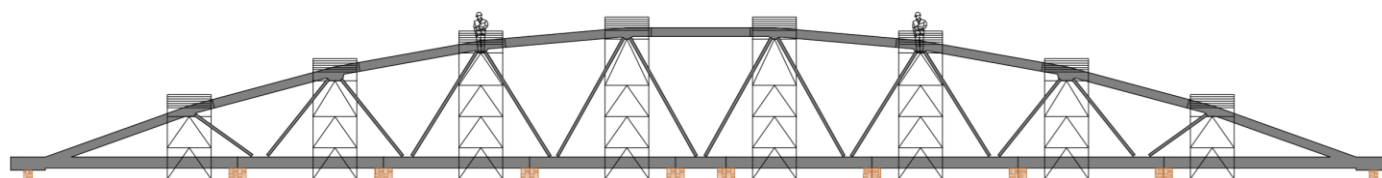
Figura 75 Tesado completo de las péndolas
