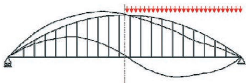
Figura 32 Ley de momentos en bowstring con péndolas verticales frente sobrecargas asimétricas [Ortega et al. 2010]
