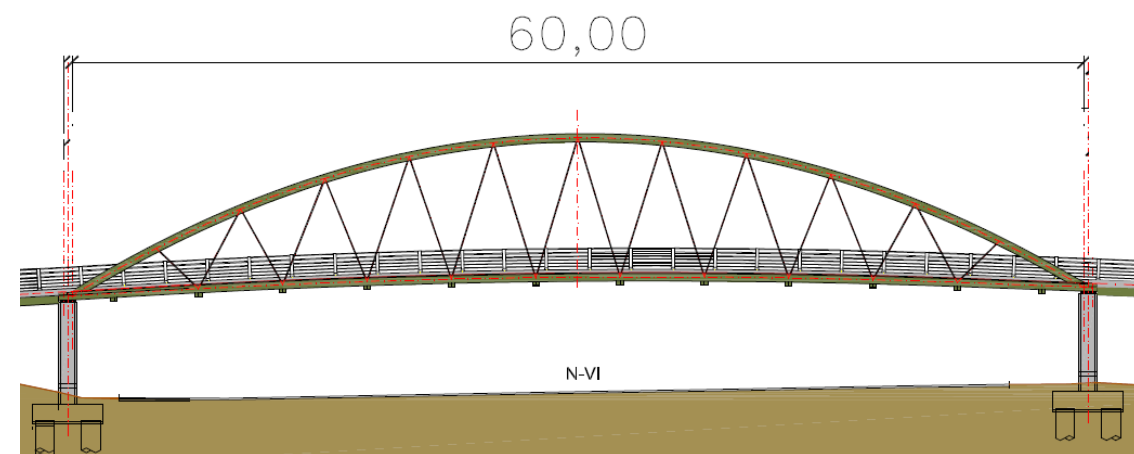
Figura 22 Vista frontal de la pasarela del Anillo Verde Ciclista de Madrid sobre la N-VI [Millanes 2008]
