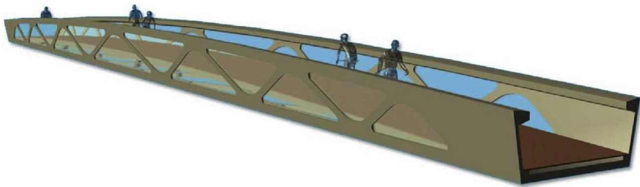
Figura 11 Vista 3D de la pasarela sobre el Barranco de las Ovejas [Serna et al. 2015]
