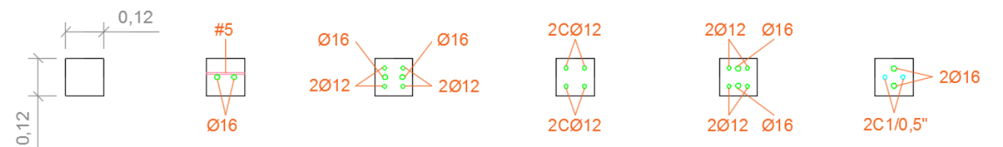
Figura 50 Secciones tipo de la péndola
