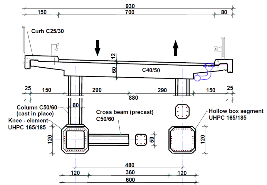
Figura 13 Sección transversal del puente en su vano central [Reichel, Sparowitz, Freytag 2011]
