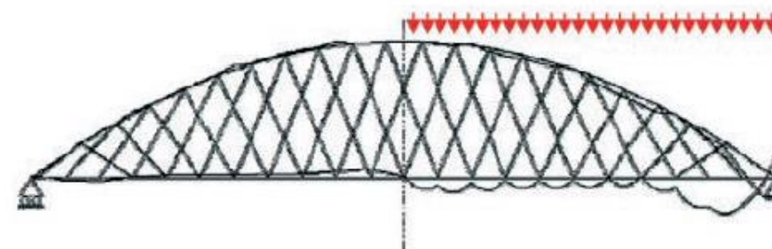
Figura 34 Ley de momentos en bowstring con péndolas inclinadas frente sobrecargas asimétricas [Ortega et al 2010]
