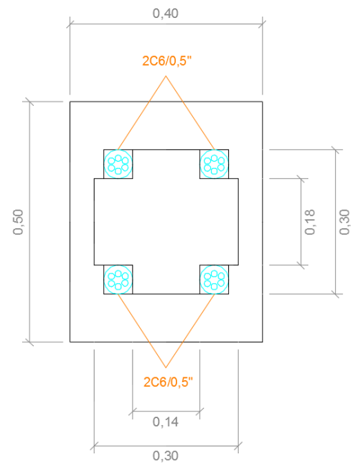
Figura 55 Sección tipo de la viga longitudinal en tramo con recrecido
