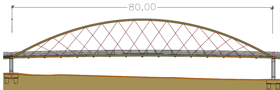
Figura 23 Vista frontal de la pasarela del Anillo Verde Ciclista de Madrid sobre la N-II [Millanes 2008]
