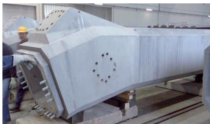
Figura 16 Elemento de unión o elemento knee [Reichel, Sparowitz, Freytag 2011]
