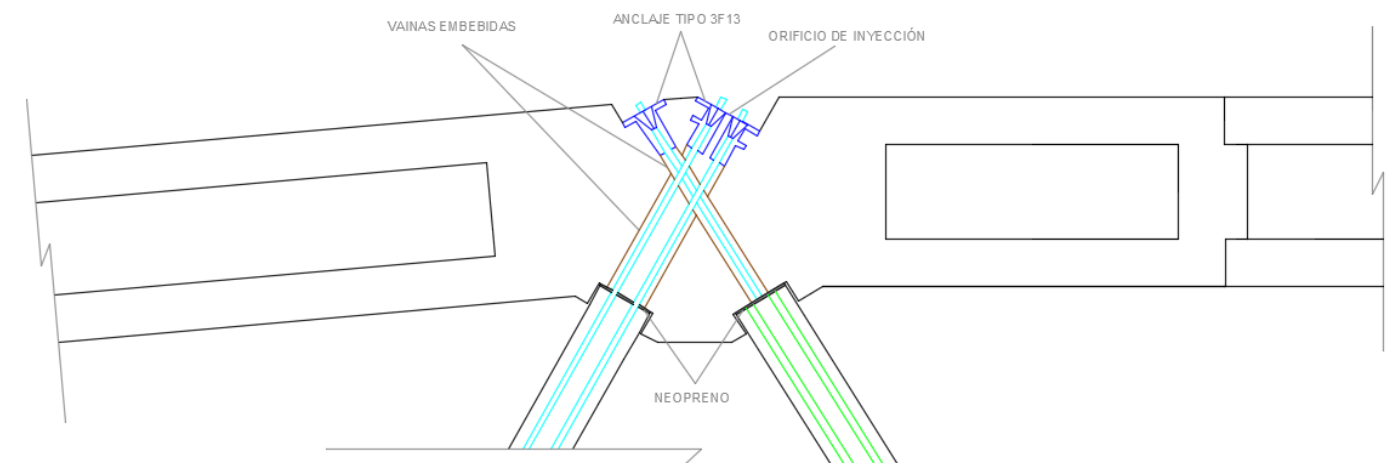
Figura 57 Detalle de unión péndola - arco
