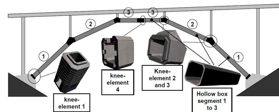
Figura 14 Resumen de elementos que forman el arco del vano central [Tue 2013]
