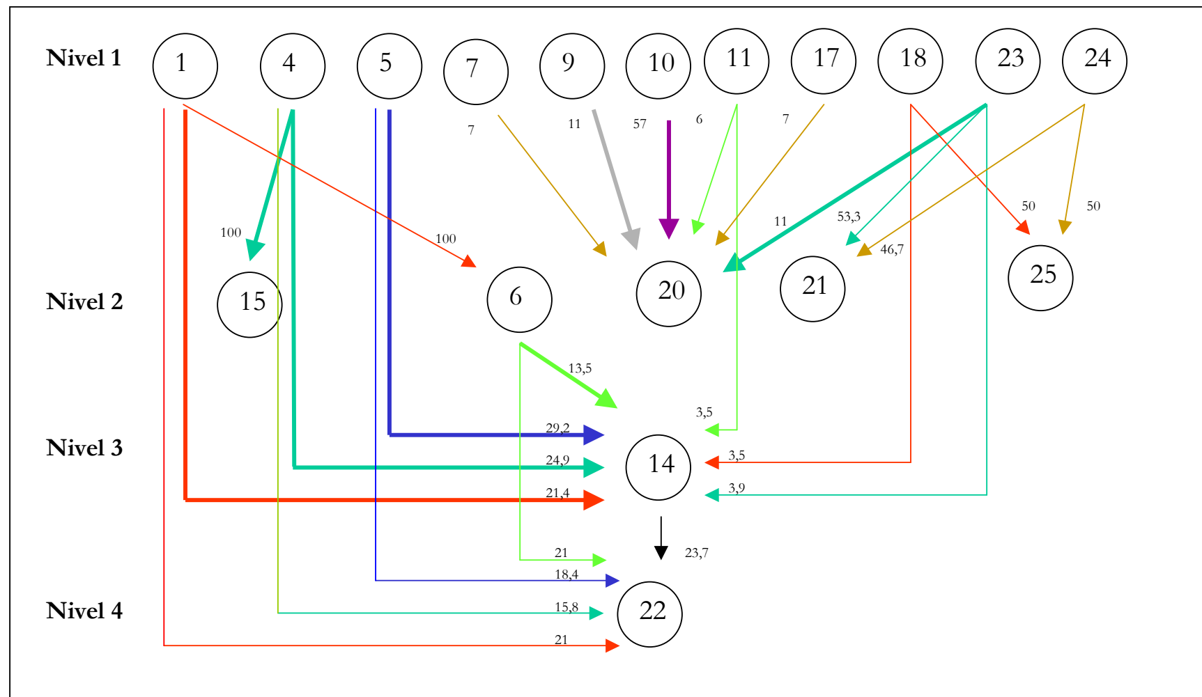
Figura 1. Grafo jerárquico J5, derivado del grafo G5
