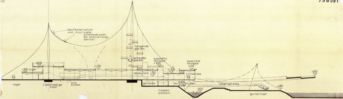
A - A schlüssel siehe lageplan
