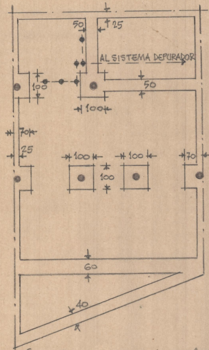
Planta de cimentación y desagües
