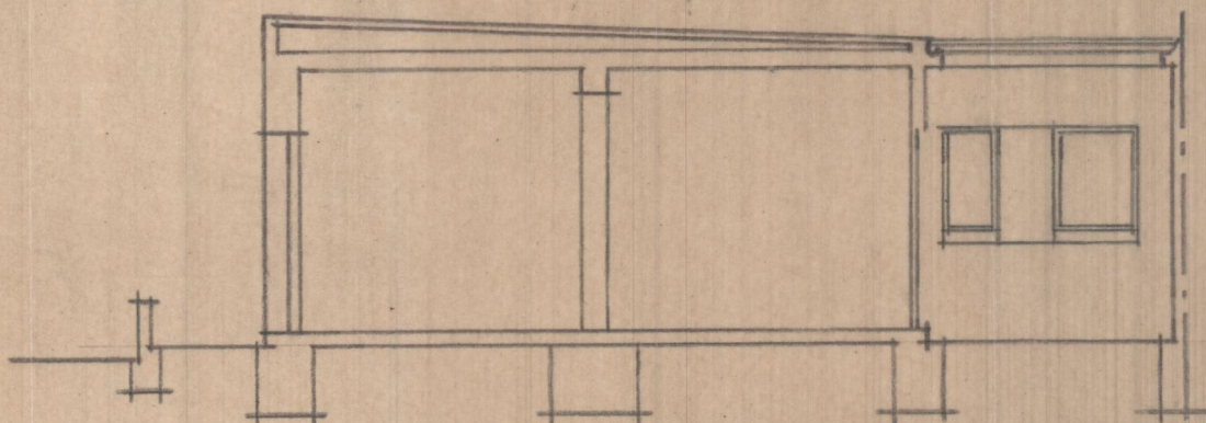
Sección por el eje
