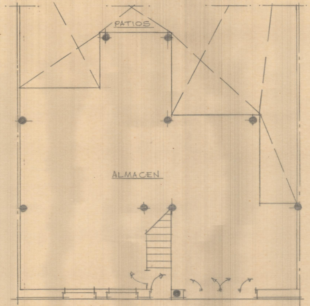
Planta baja definitiva
