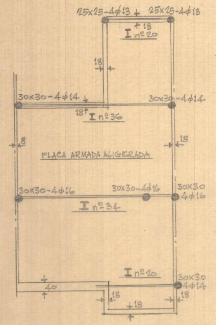
Estructura de cubierta
