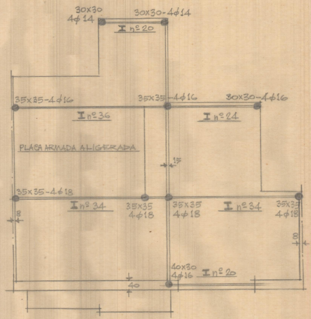
Estructura de fijo
