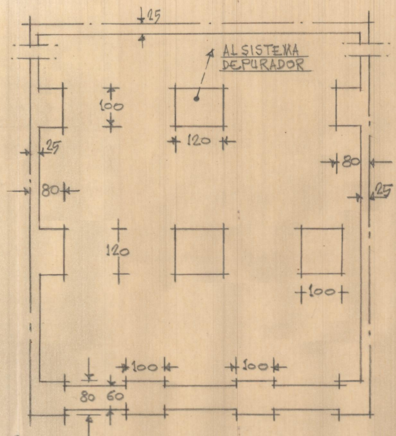
Planta de circunferencia de desagües
