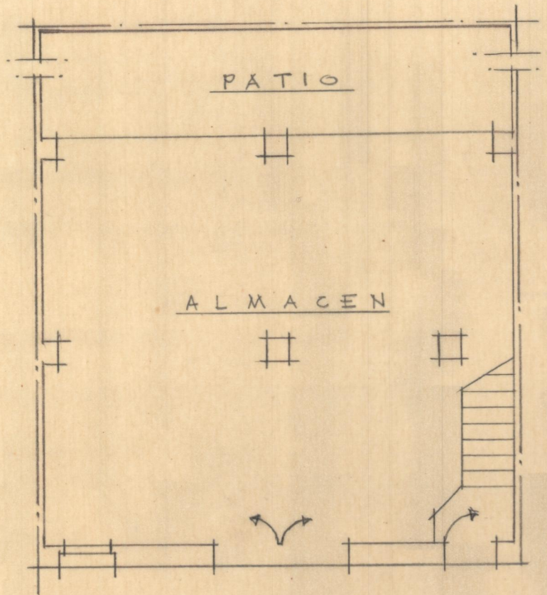
Distribución en planta baja
