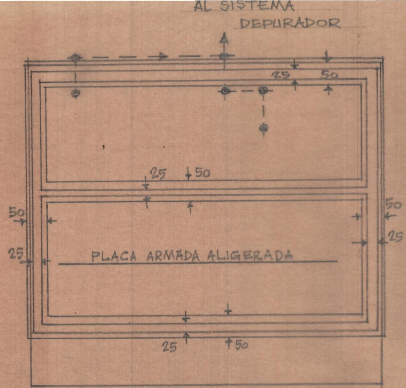
Cimientos y cubierta de drenaje
