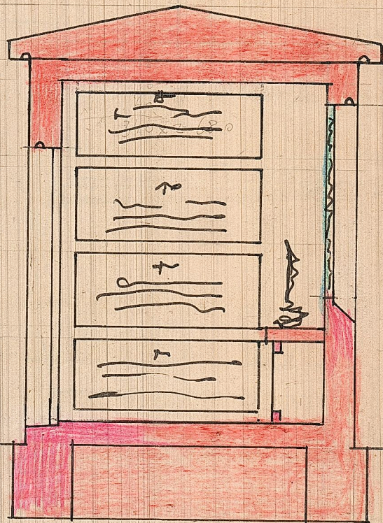
SECCION LONGITUDINAL
