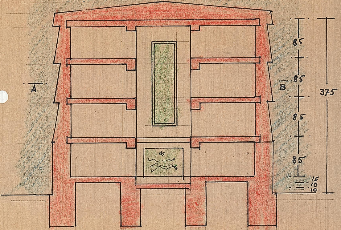
SECCION TRANSVERSAL
