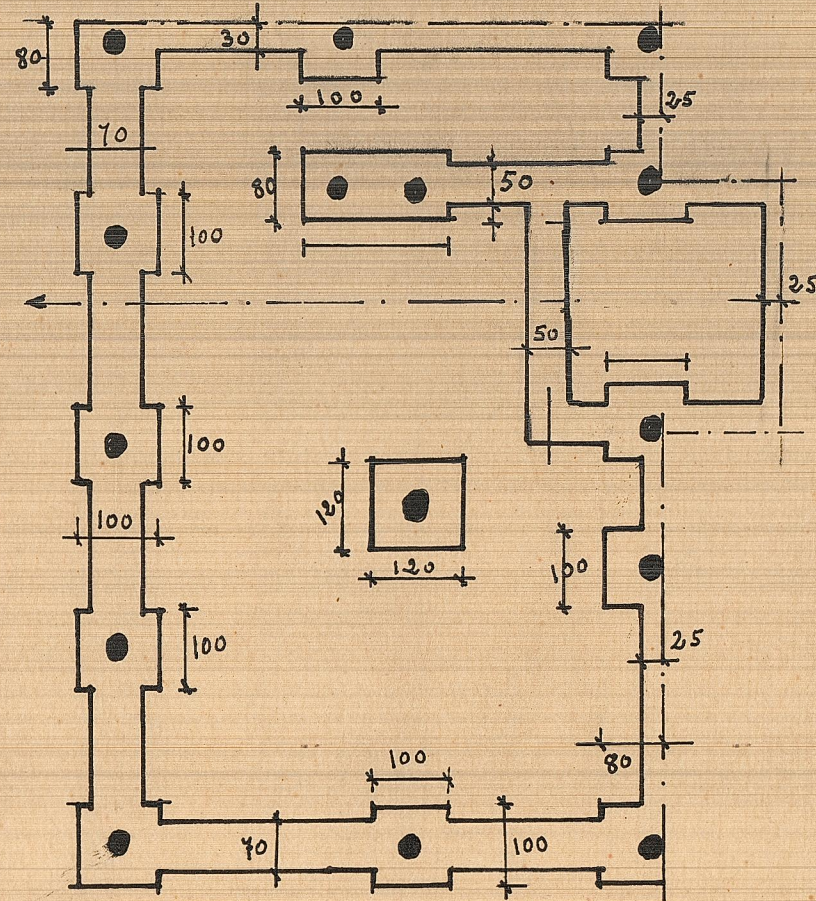
Planta de cimientos y desagues
