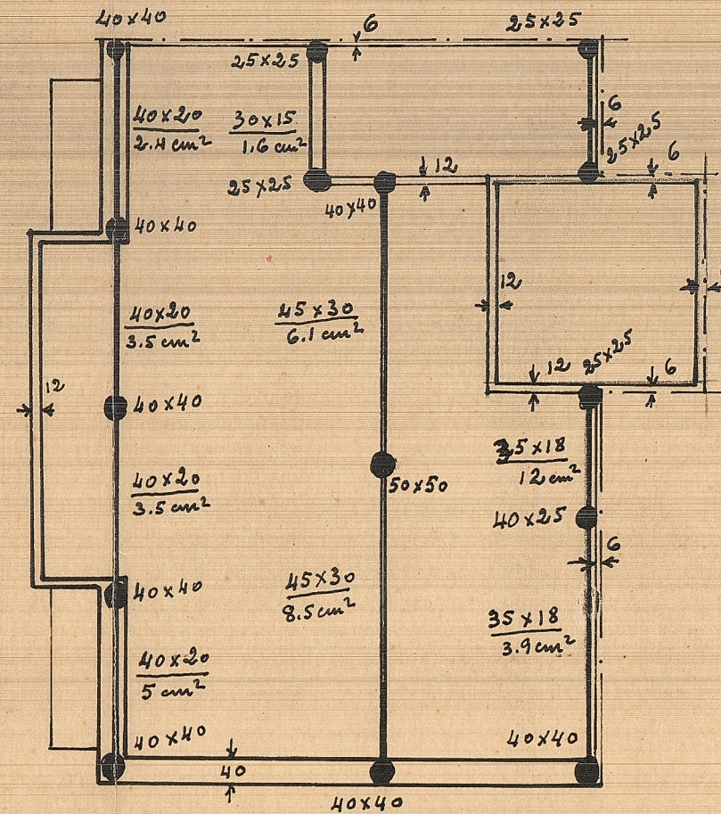
Estructura de pisos y cubierta
