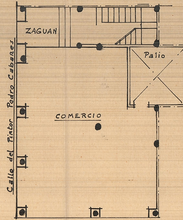
Disposición en planta baja
