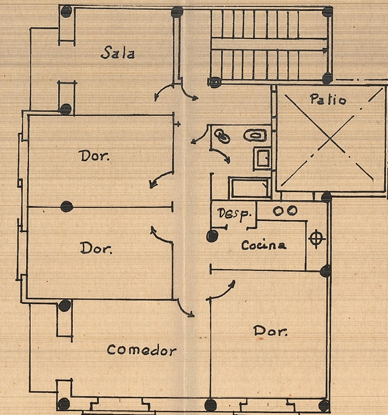
Disposición en plantas altas
