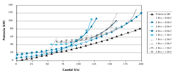
Fig. 5. Evolución de la potencia útil y la potencia absorbida por la estación de bombeo con el caudal. (Bvv = Bomba de velocidad variable; Bvf = Bomba de velocidad fija)
