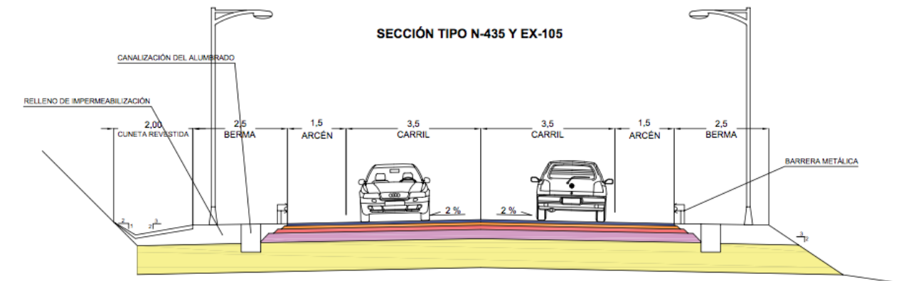
Figura 40. Sección tipo de N-435 y EX-105. Elaboración propia con AutoCad.
