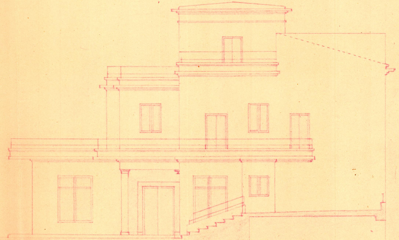
FACHADA LATERAL
