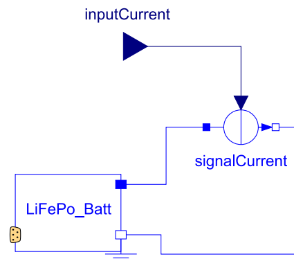
Figura 8: Modelo para calibración con entrada de intensidad de descarga
