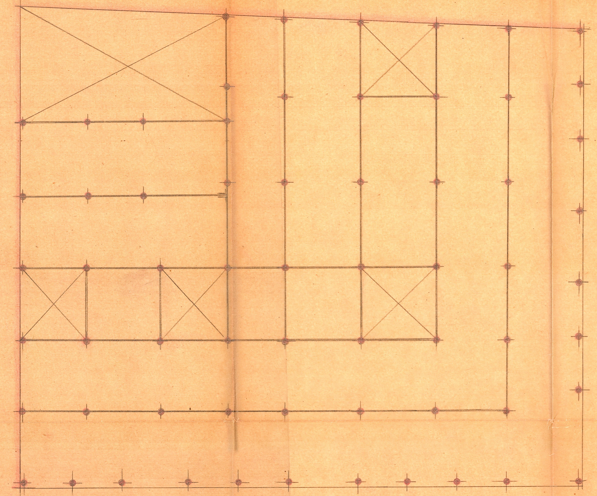
Planta de pilares y entramado
