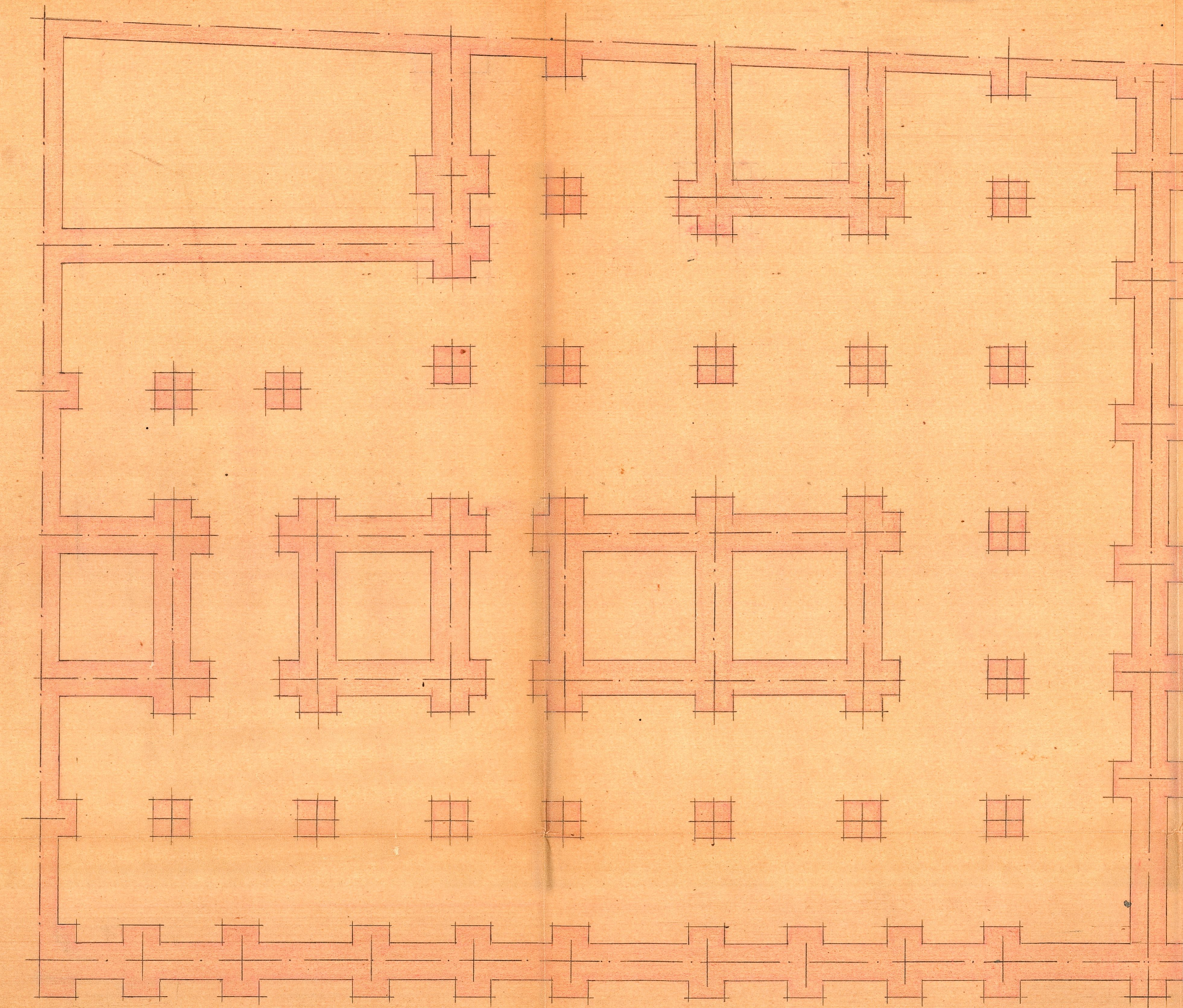
Planta de cimientos
