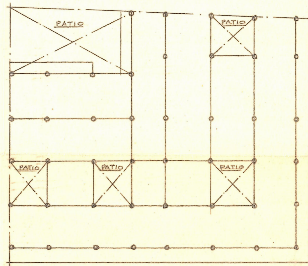
Entramado de la cubierta del ático
