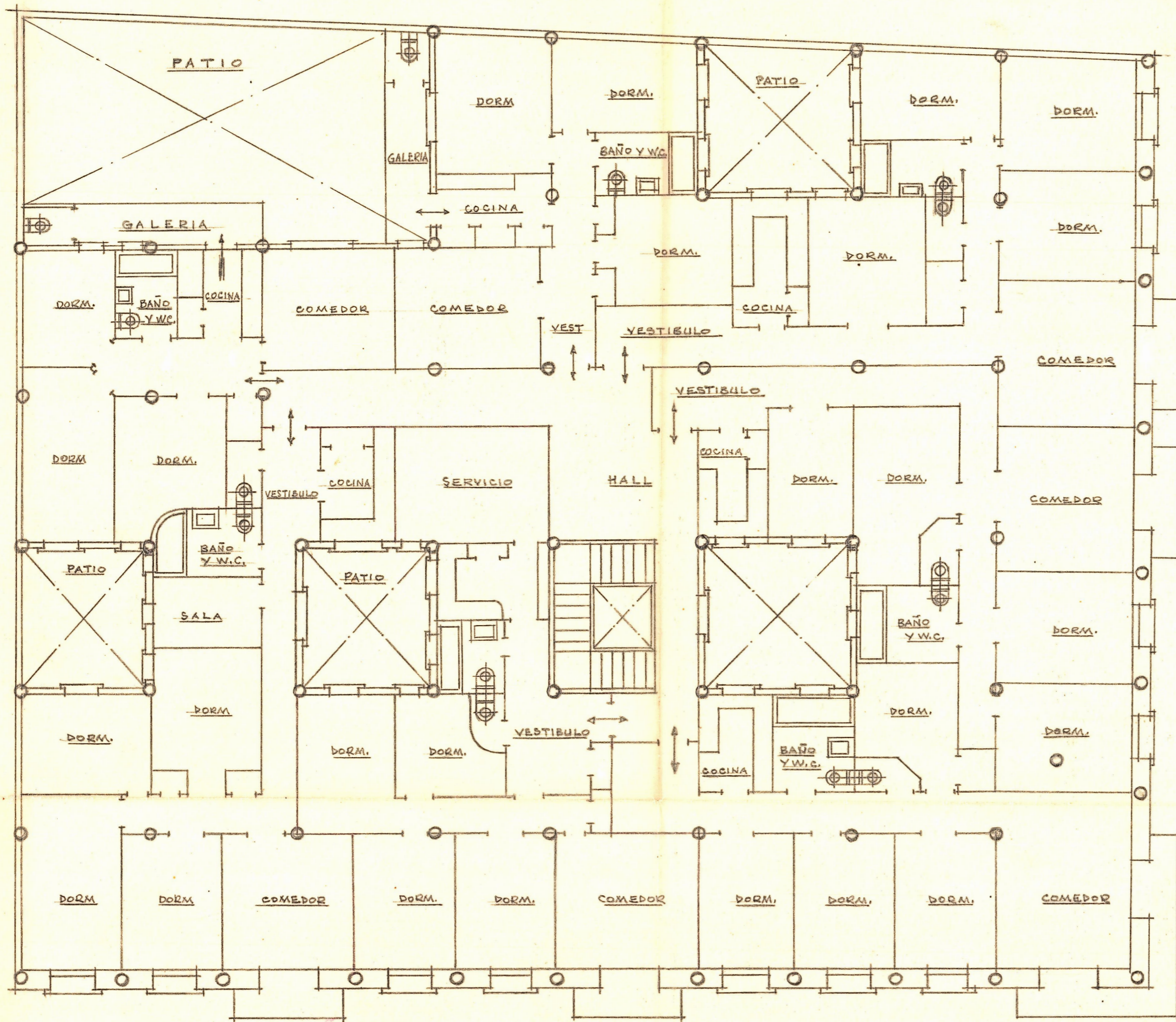
Planta con las medidas
