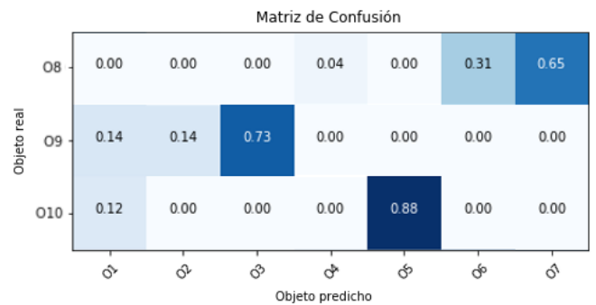
Figura 10: Matriz de confusión para el modelo MLP 3st entrenado con DS-I y evaluado con DS-III usando el descriptor raw .
