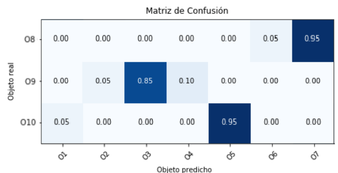
Figura 11: Matriz de confusión para el modelo MLP 3st entrenado con DS-I y evaluado con DS-III usando el descriptor diferencial .
