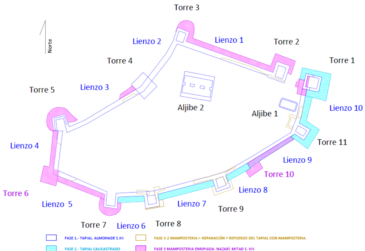
FASES CONSTRUCTIVAS DEL CASTILLO DE PÍÑAR. FASES I + ii + III
