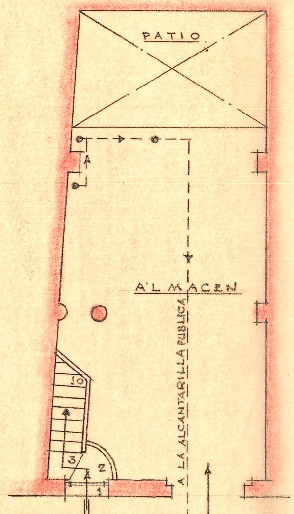
Planta baja y delagües
