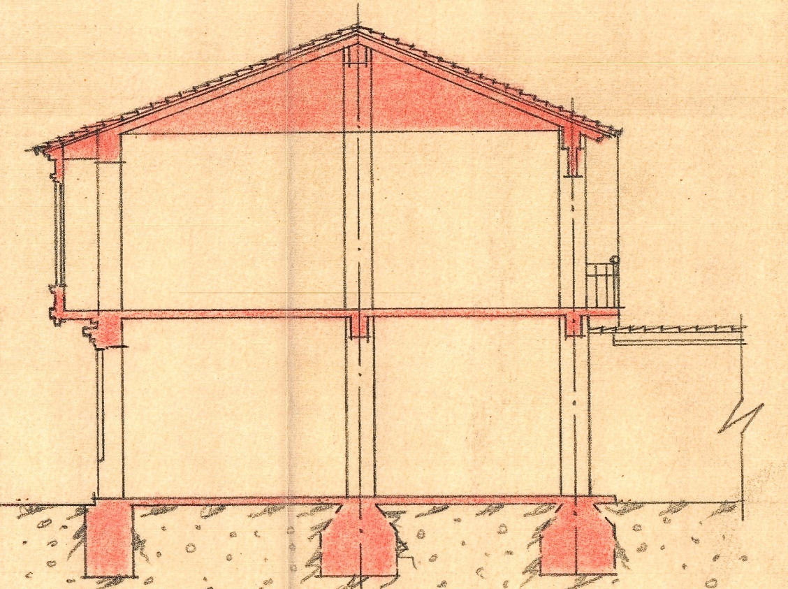
Sección longitudinal
