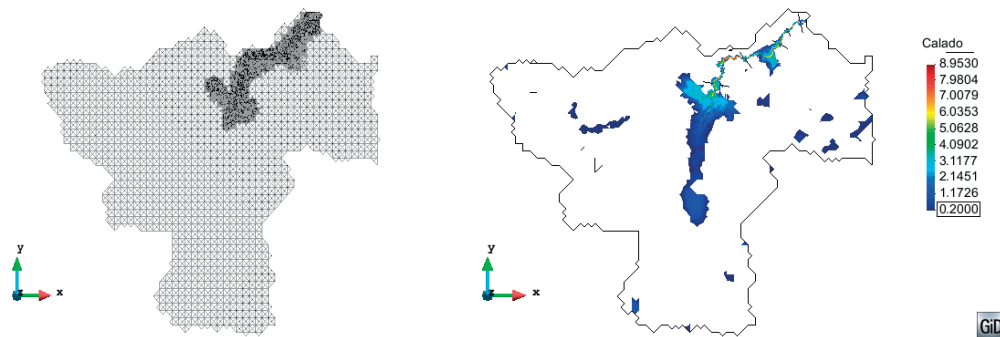
Figura 4 | Malla de cálculo (izquierda) y mapa de inundabilidad (derecha) para la cuenca de cabecera del río Fluvità realizado mediante modelización integrada hidráulico-hidrológica.
