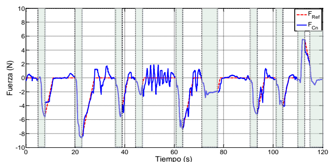
Figura 9: Ensayo en modo activo en la configuración mecánica ARM. Con el fondo verde se destaca el movimiento de flexión.
