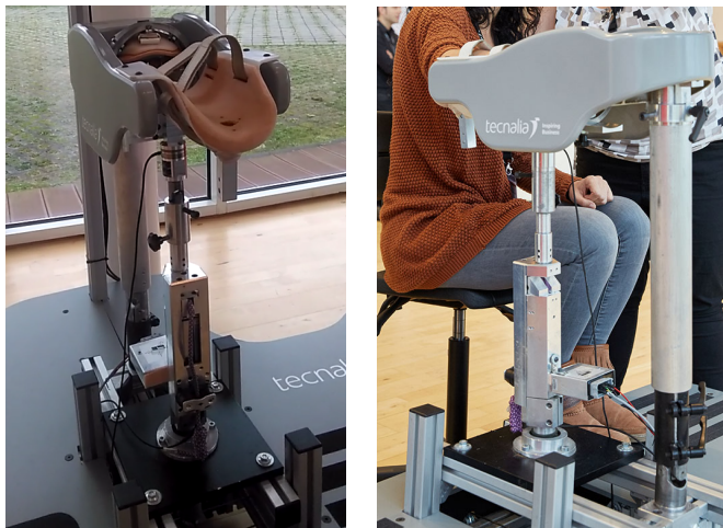
Figura 2: El robot de rehabilitación UHP (Universal Haptic Pantograph) sin y con usuario.
