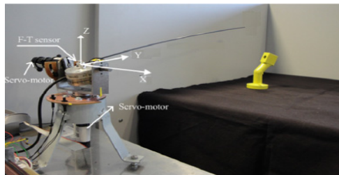
Figura 4: Plataforma experimental.
