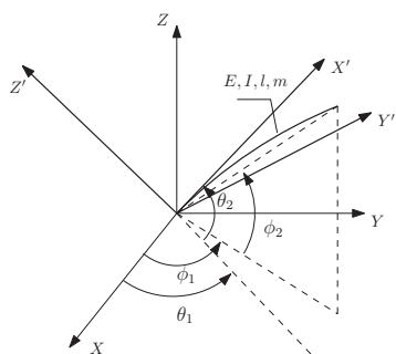
Figura 6: Modelo esquemático de la antena sensora
