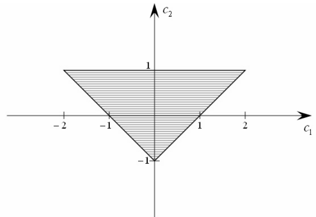
Figura 2: Área de estabilidad de la ecuación característica como una función de los parámetros c_1 y c_2 .
