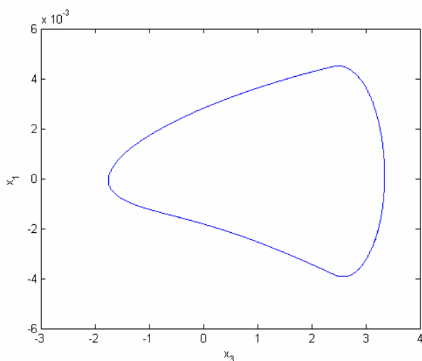
Figura 10. Retrato de fases del atractor derecho de González estabilizado en torno a una UPO correspondiente al parámetro R = 24 K\Omega .
