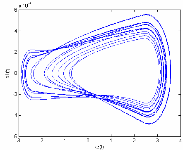
Figura 7: Retrato de fases del atractor de González para los parámetros R_L = 0,09 K\Omega , R = 18,5 K\Omega , A = 5,8 y condiciones iniciales x_1(0) = 0 A , x_2(0) = 3 V y x_3(0) = 0,3 V .
