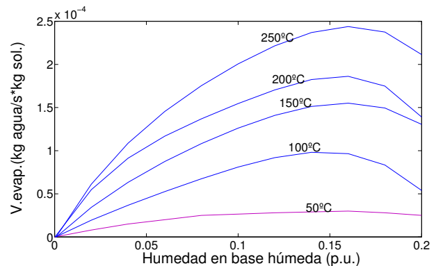
Figura 11. Velocidad de secado en función de la humedad de sólido.
