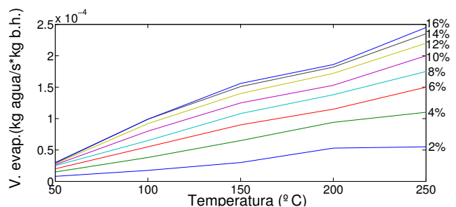
Figura 12. Velocidad de secado en función de la temperatura de gas.
