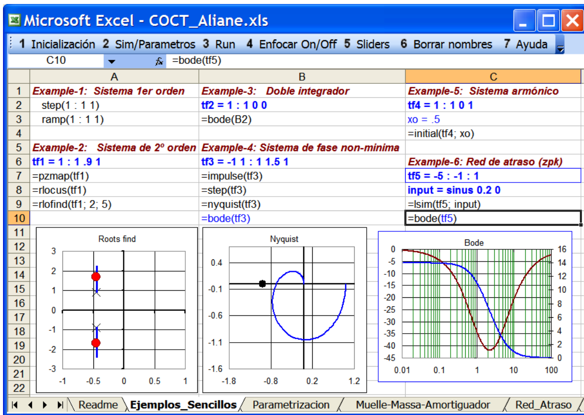
Figura 1. Aspecto general del entorno COCT.
