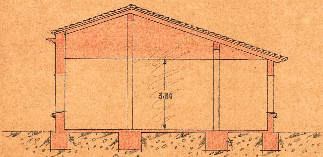
Sección transversal
