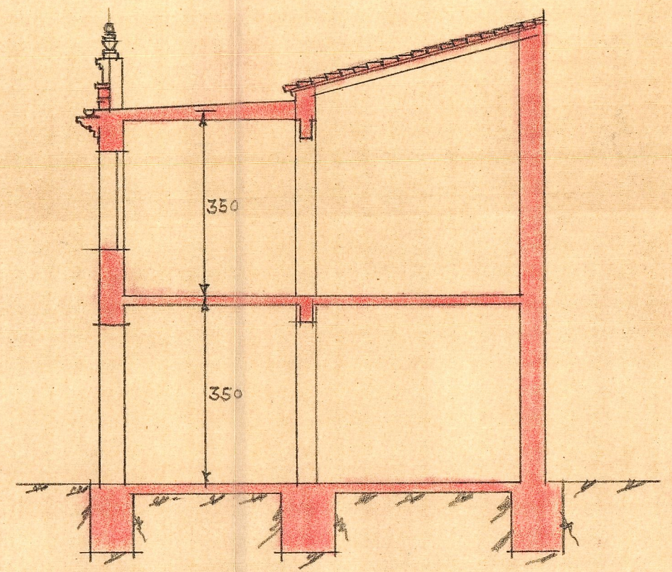
Seccion por A-B
