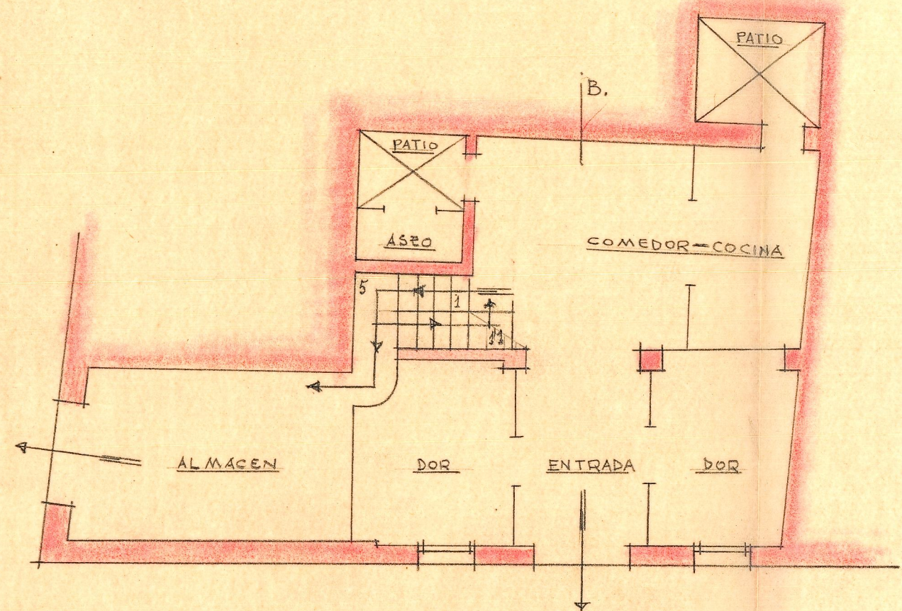
Planta baja
