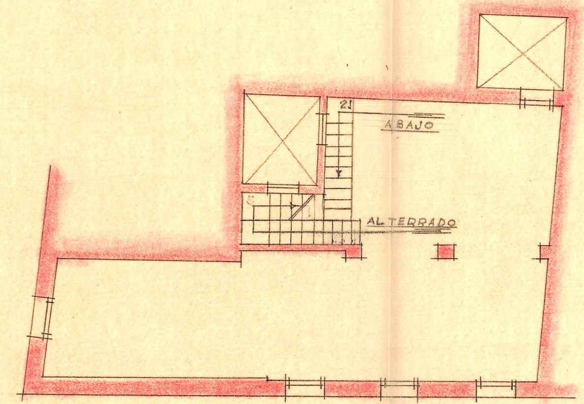
Planta alta
