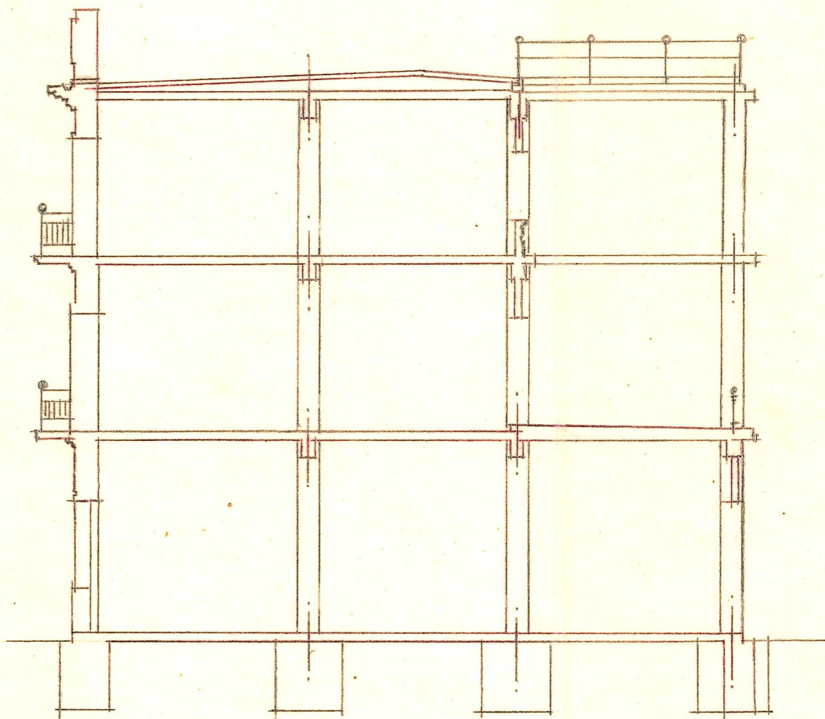
Sección por A-B
