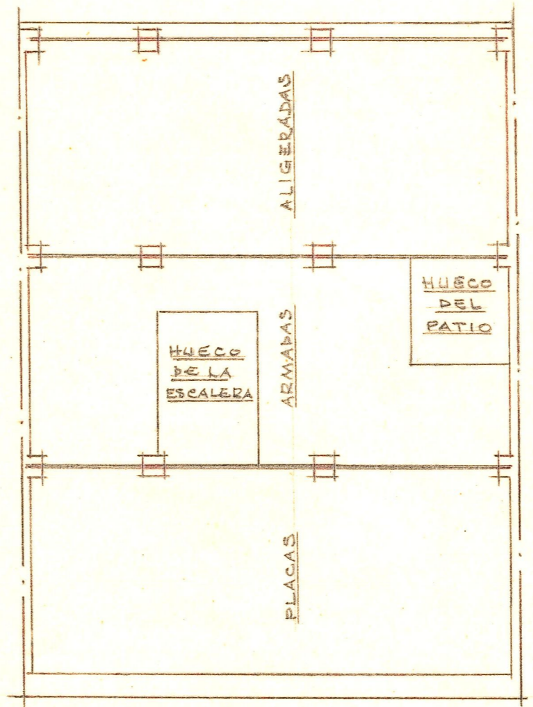
Entramado de fuste
