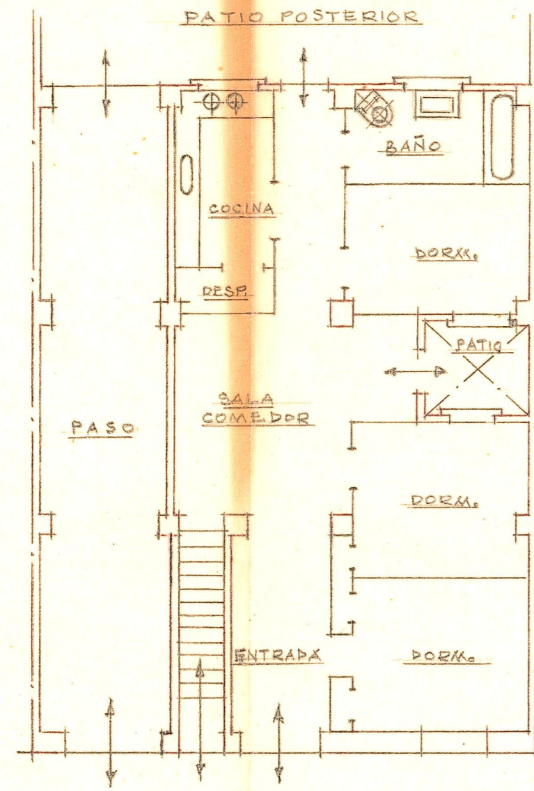
Planta baja
