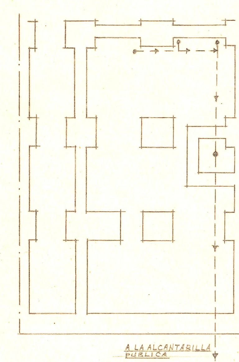
Planta de cimentación y desagües
