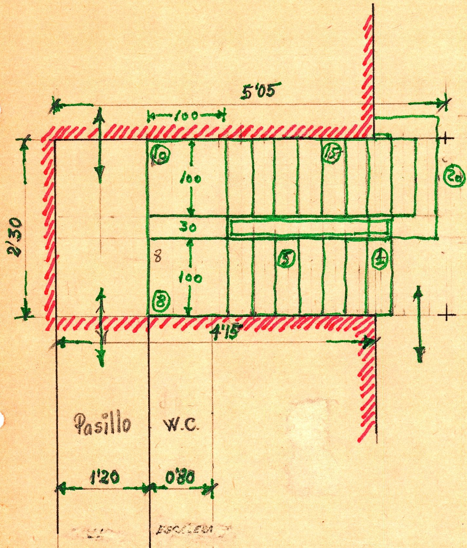
EL MICALET - ESCALERA - 3-OCTUBRE DE 1965 - ESC. - 1:50
