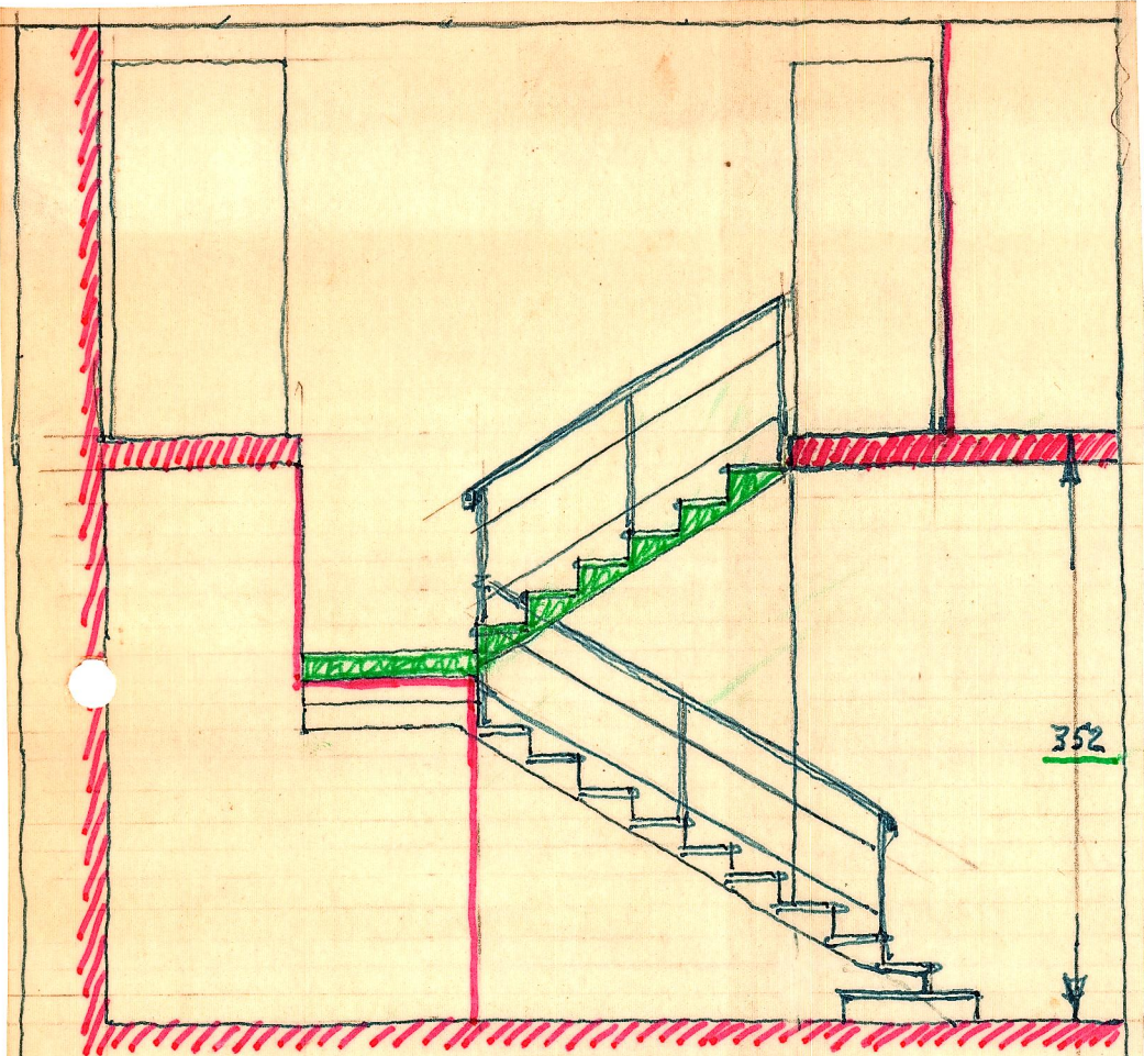
SECCION AB
