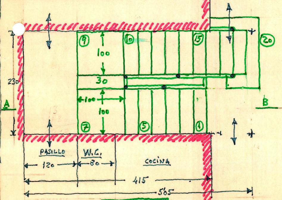
PLANTA BAJA
