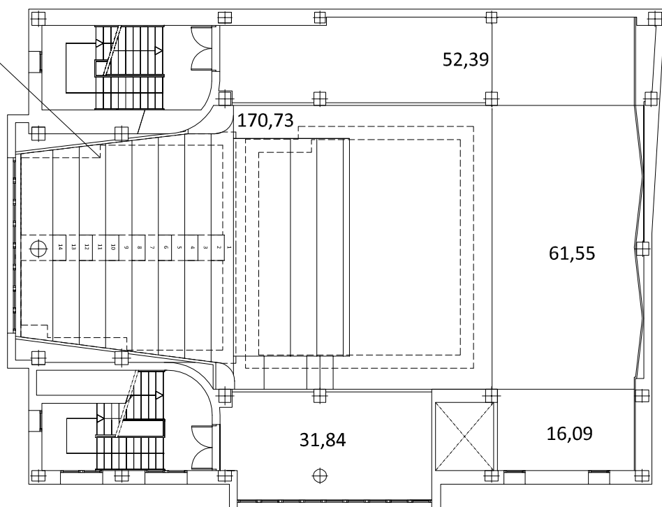
PLANTA PRINCIPAL
