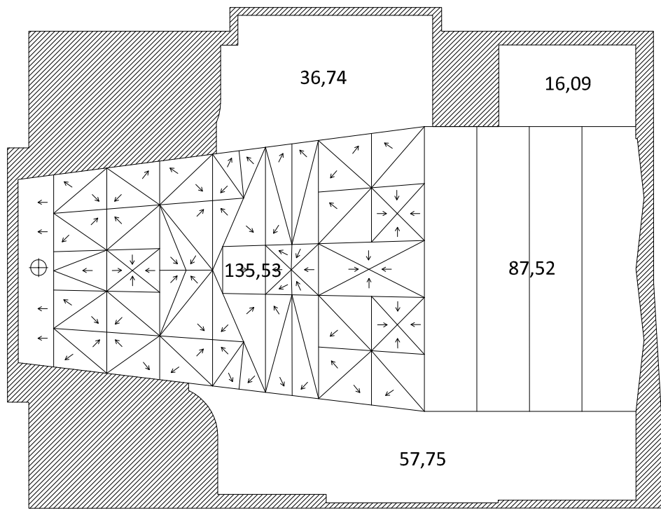
PLANTA CENTRAL
