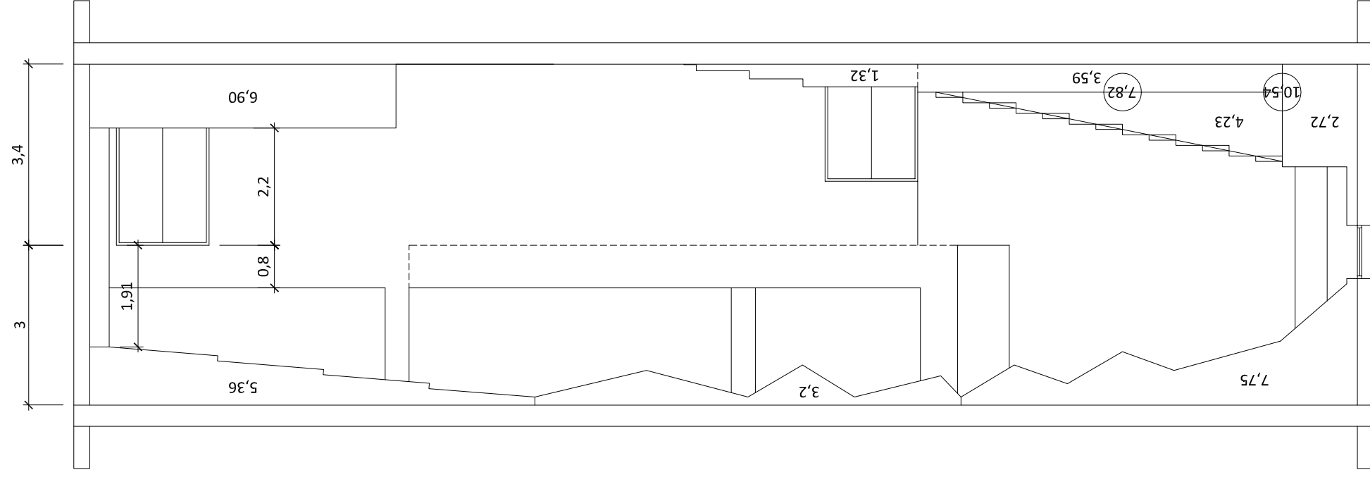
SECCIÓN LONGITUDINAL
