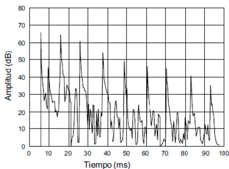
Fig. (21) Curva energía-tiempo ETC ilustrativa de la existencia de eco flotante.
