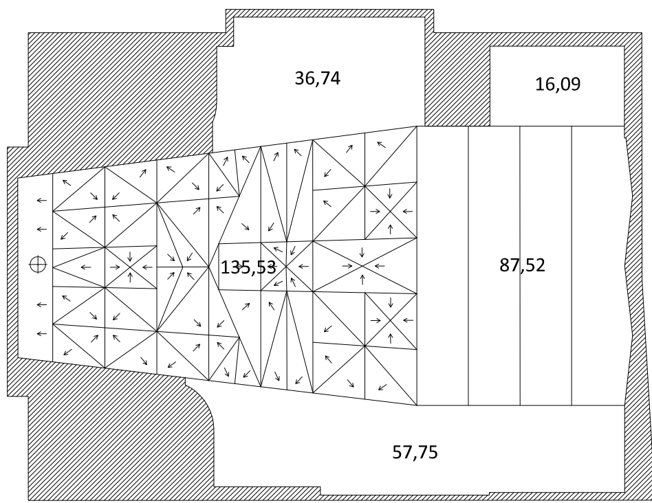
PLANTA CENTRAL
