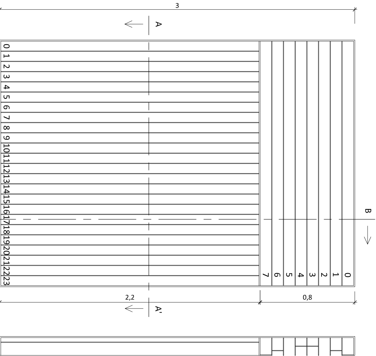
SECCIÓN B-B'
