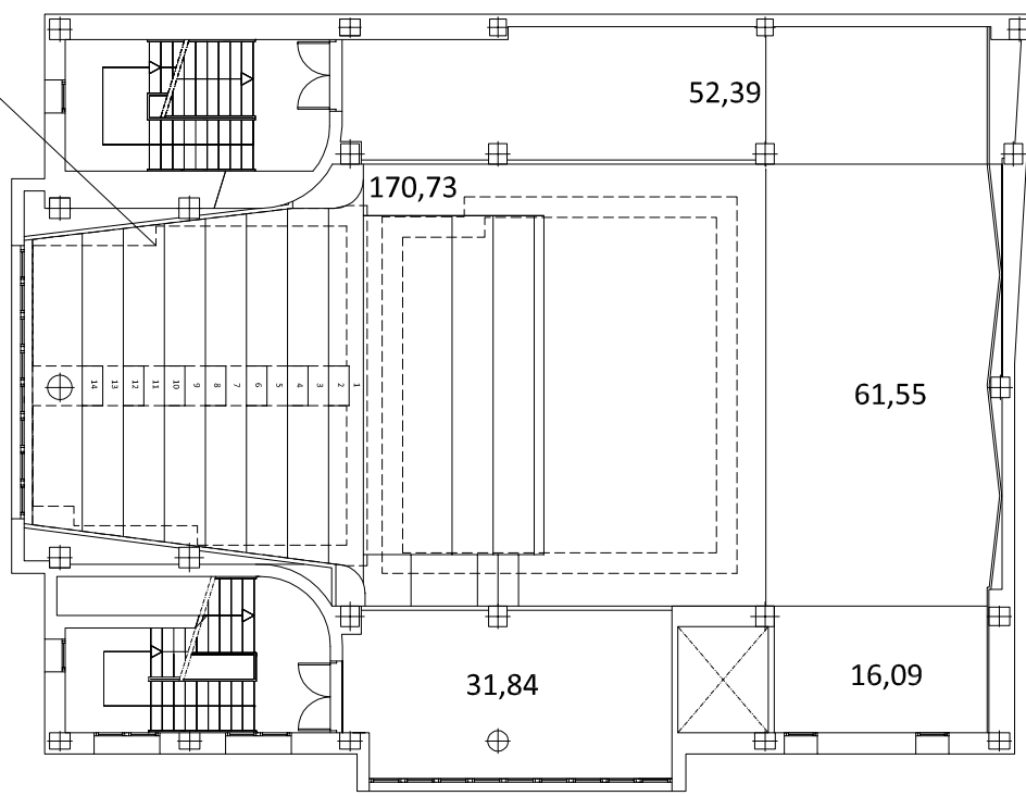
PLANTA PRINCIPAL
