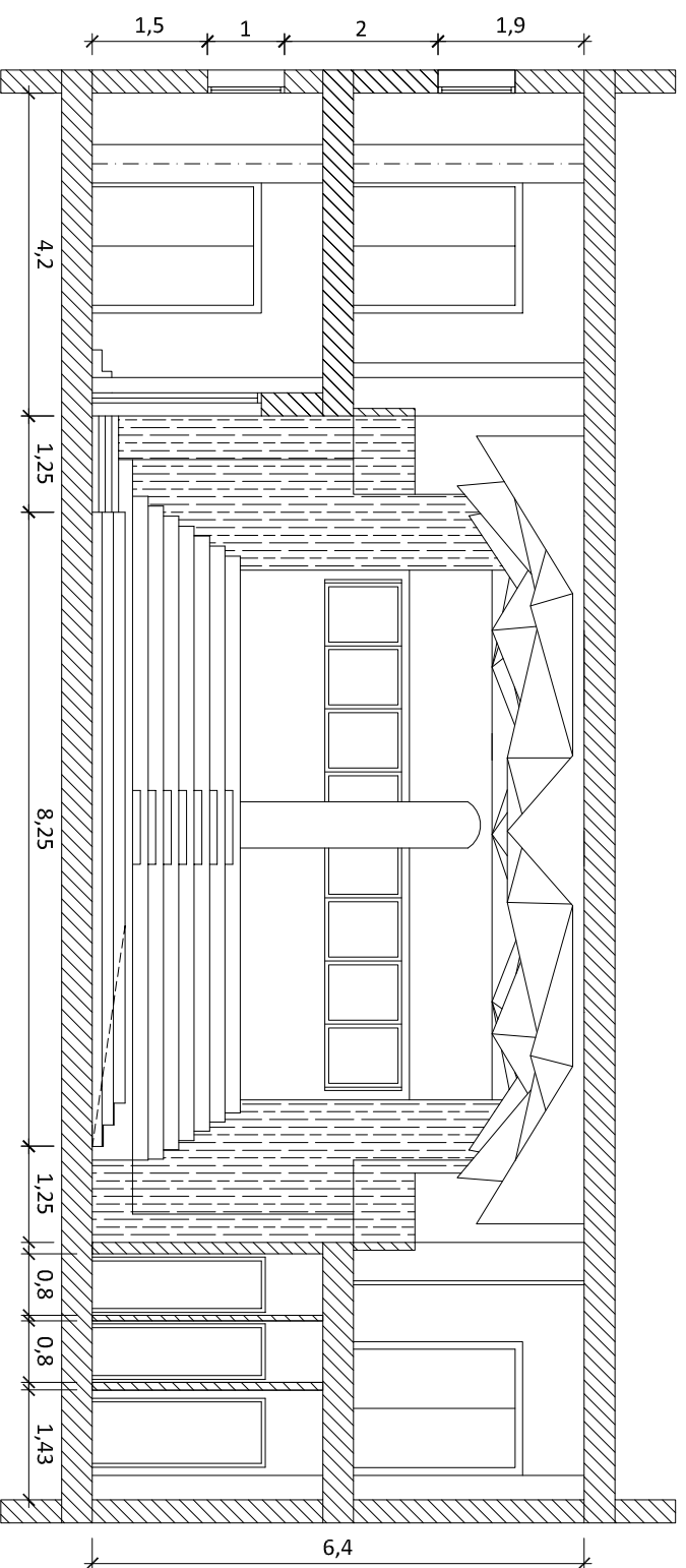
SECCIÓN C-C'
