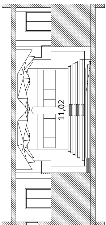
SECCIÓN TRANSVERSAL 2
