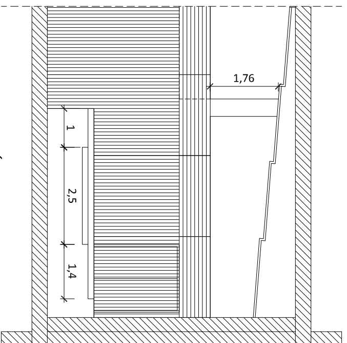
SECCIÓN B-B'
