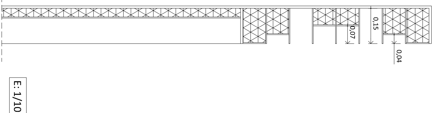
DETALLE DEL DIFUSOR EN EL PLANO VERTICAL (p=7)
