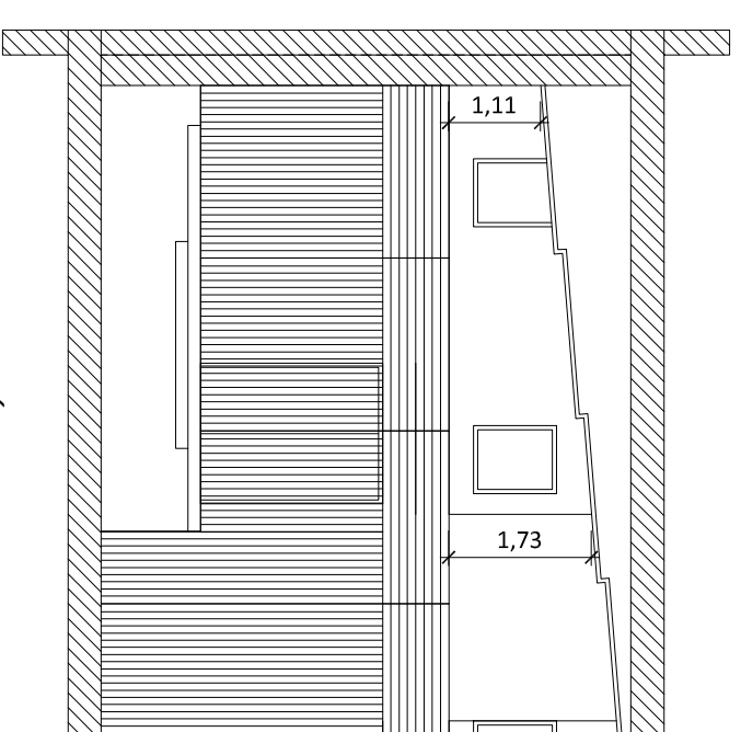
SECCIÓN A-A'
