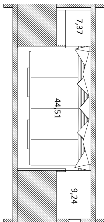
SECCIÓN TRANSVERSAL 1
