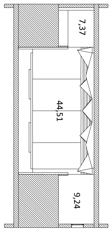
SECCIÓN TRANSVERSAL 1
