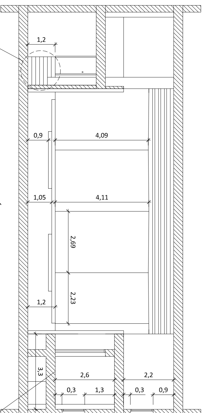
SECCIÓN VERTICAL
