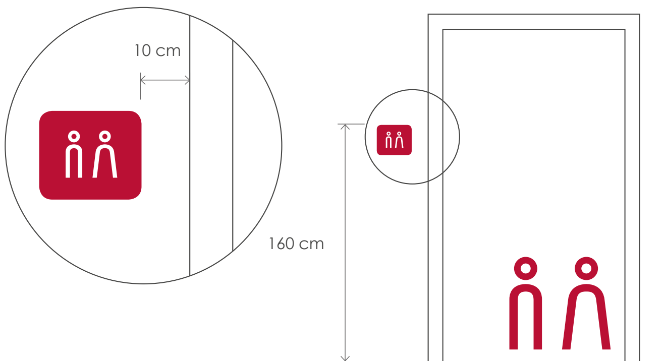
Altura máxima señal principal y separación del marco de la puerta.
