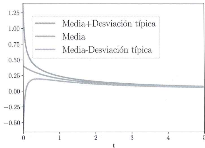
Figura 1: Gráficas de la función media y de la media más/menos una desviación típica del proceso estocástico solución en el contexto del ejemplo.
