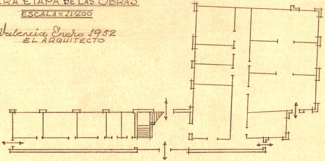
Planta baja
