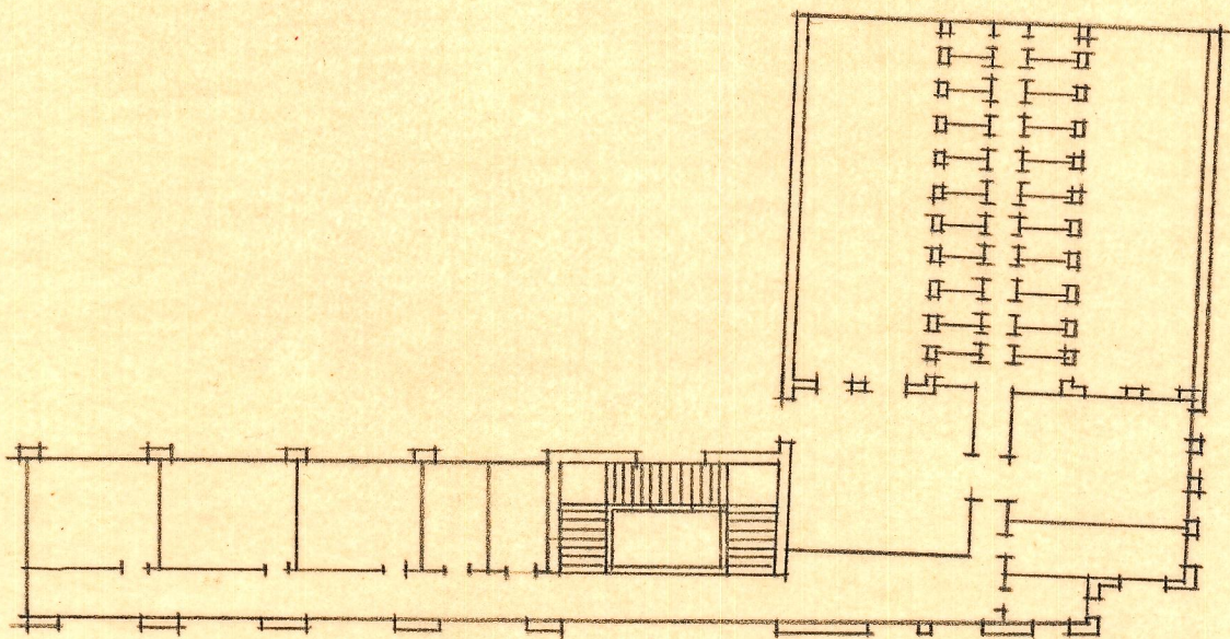
Piso Segundo
