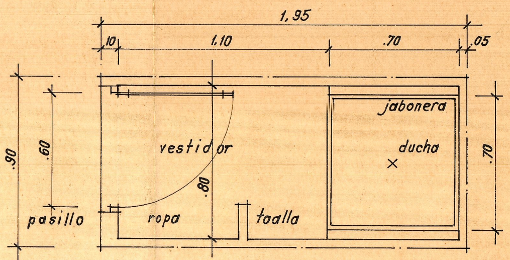
planta de una ducha (esc. 1:20)
