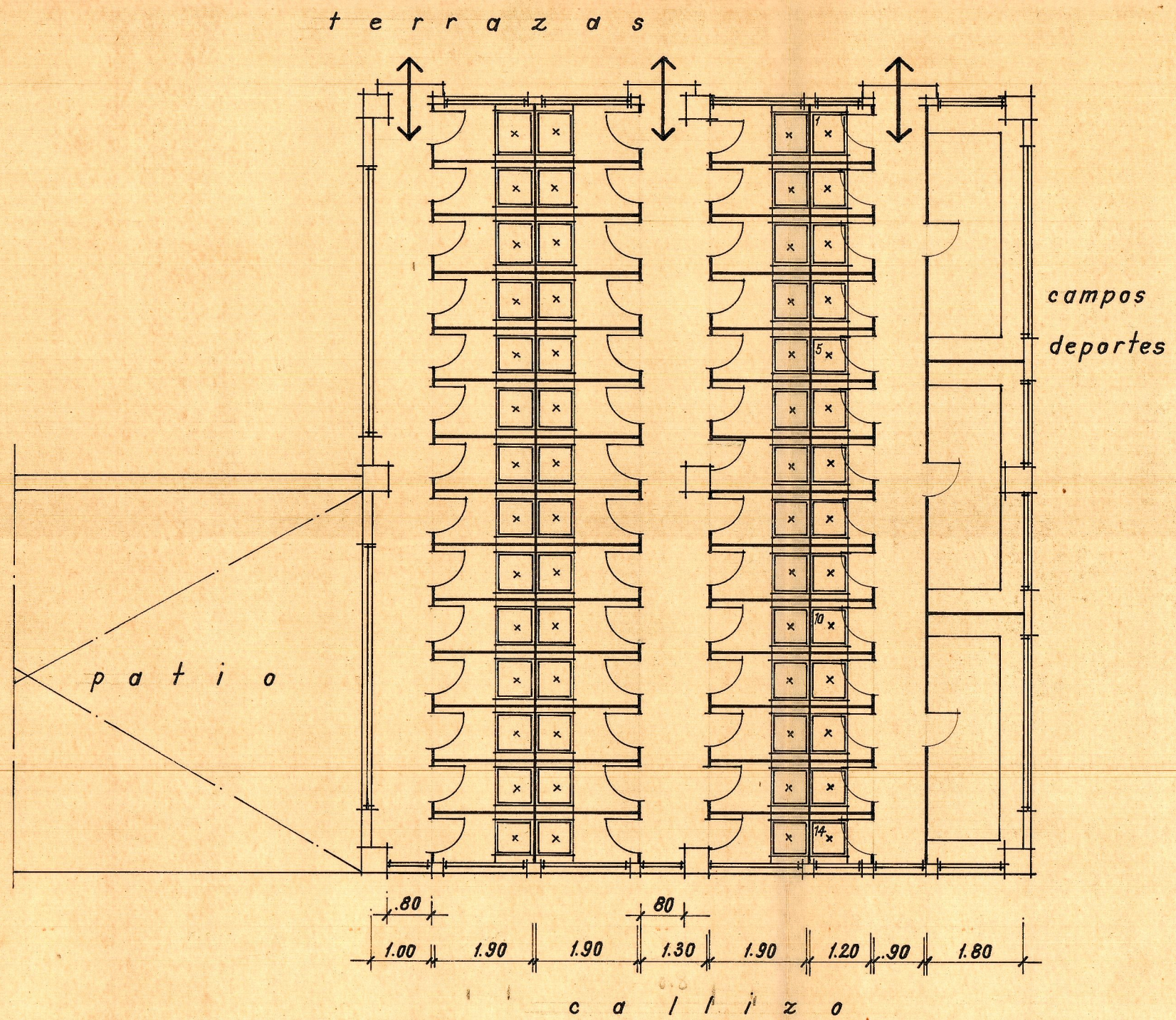
duchas y vestuarios esc. 1:100.
