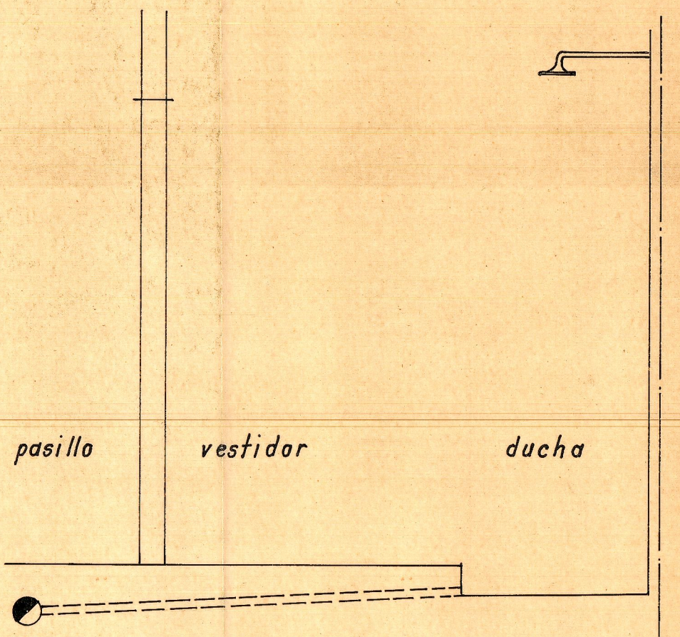
sección de una ducha (esc. 1:20)
