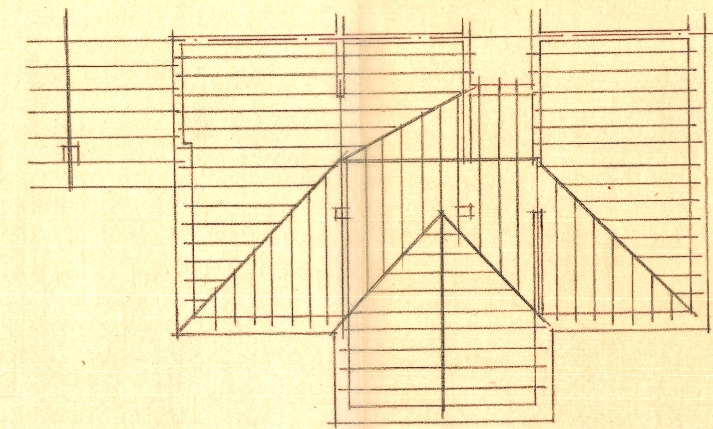
Enramados de cubierta y enlucido alto
