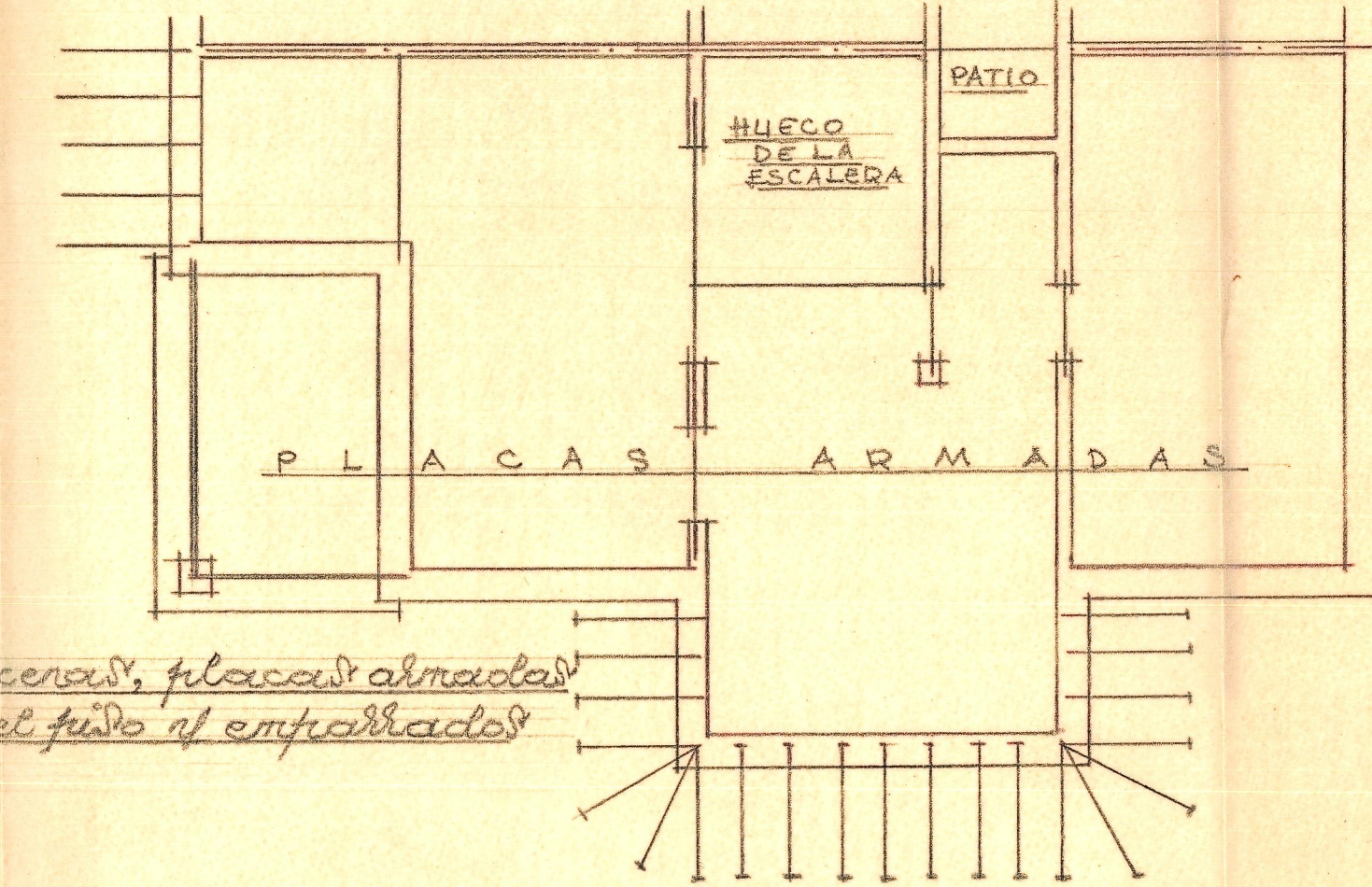
Planta de columnas y de vigas
