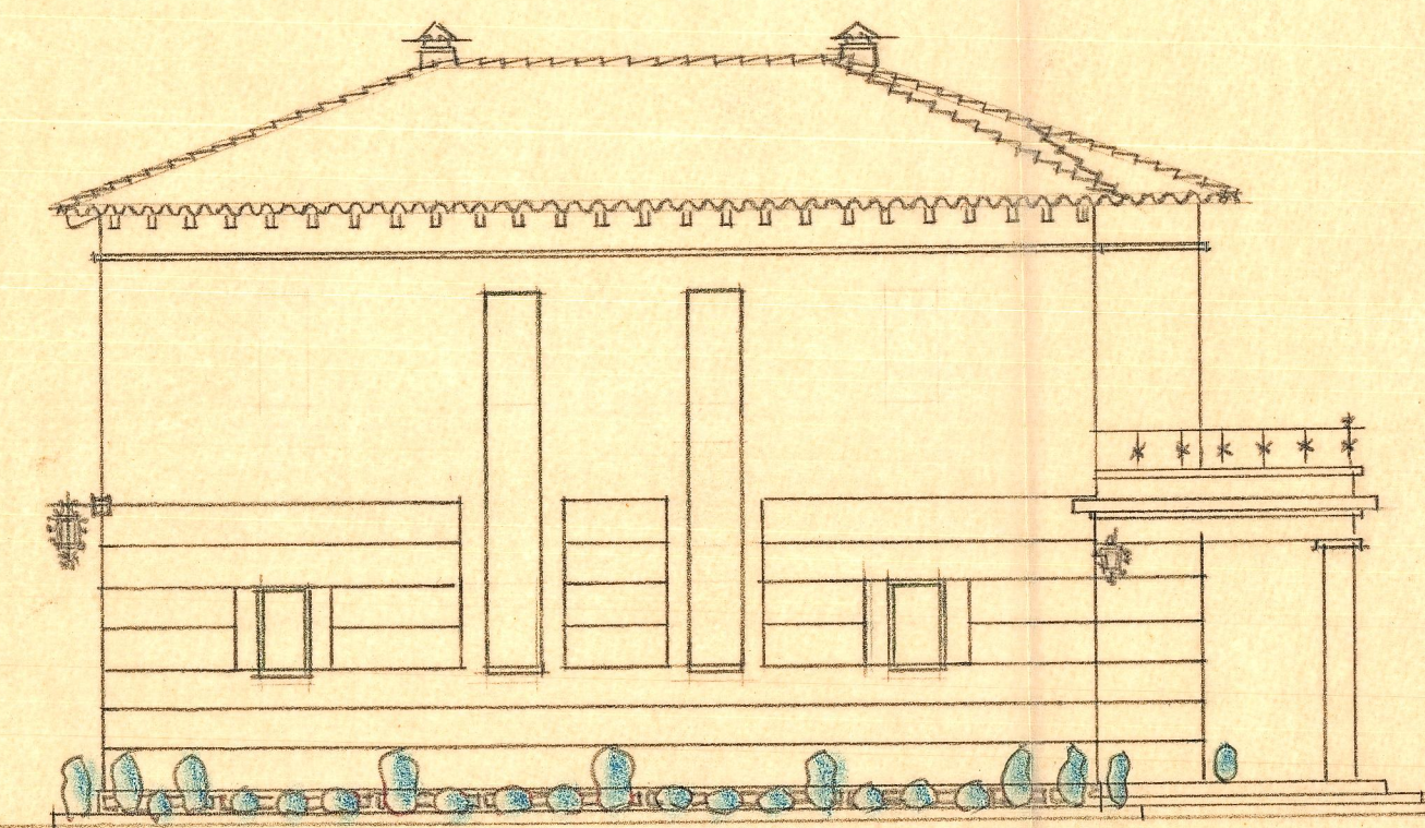
Fachada Oeste
