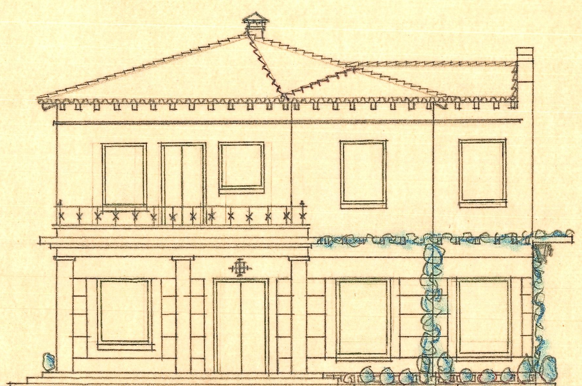
Fachada Sur
