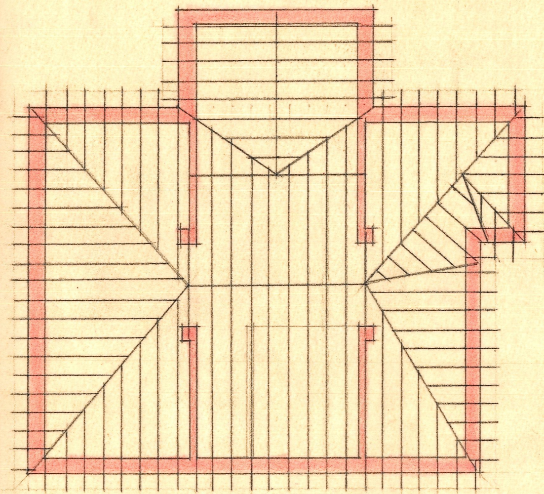
Entramado de cubierta.
