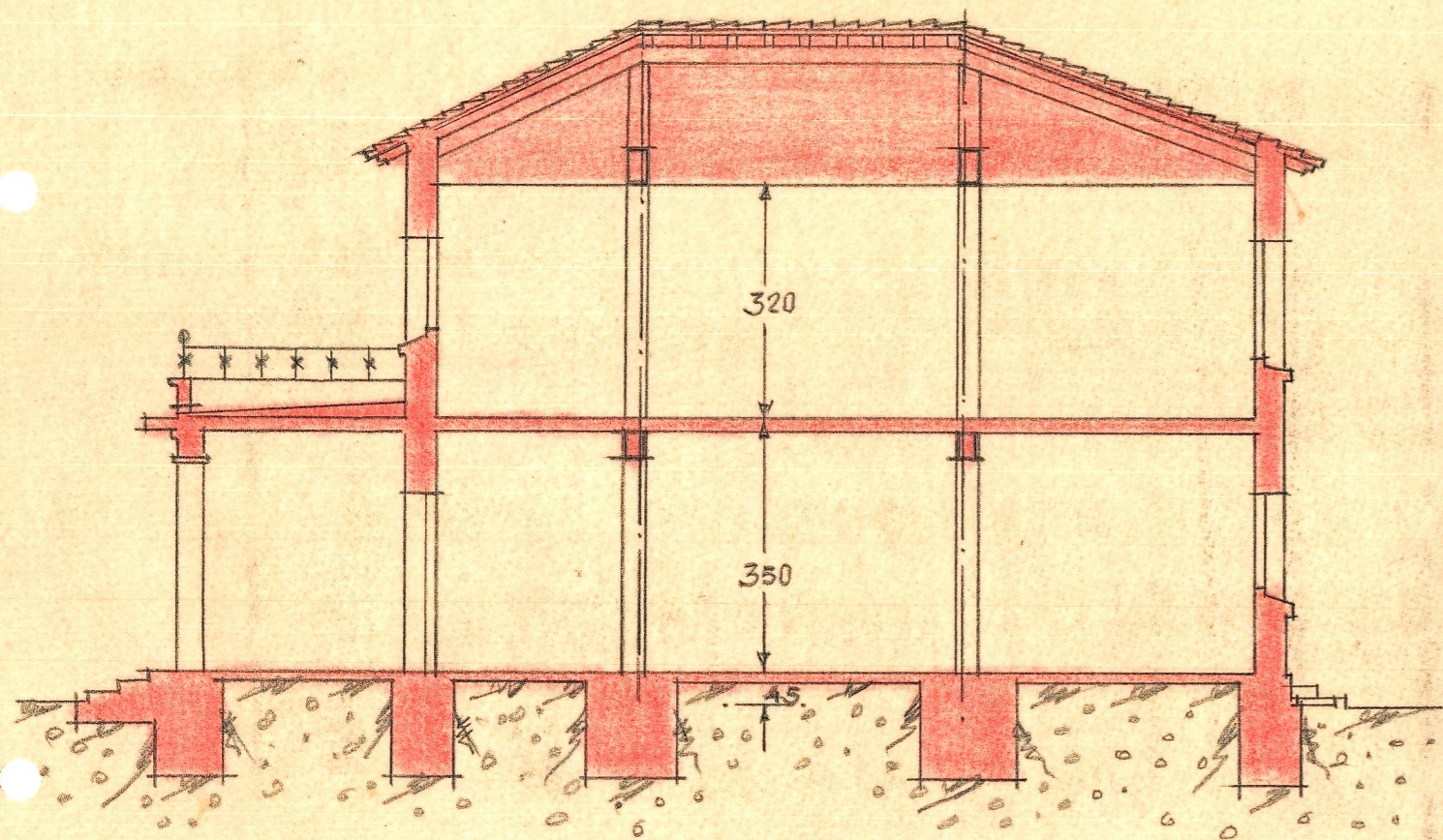
Sección longitudinal.
