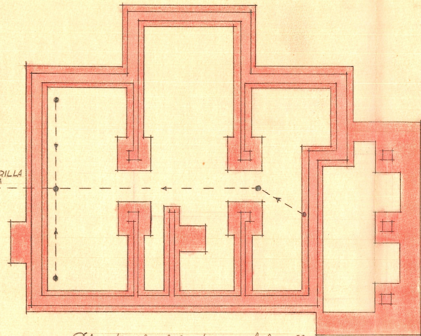
Planta de cimientos y desagües.
