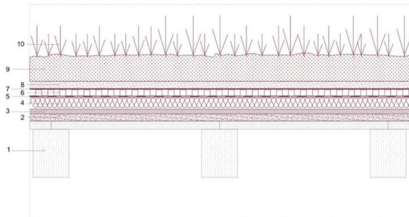
Detalle 1. Definición constructiva Cubierta 1. Elaboración propia
