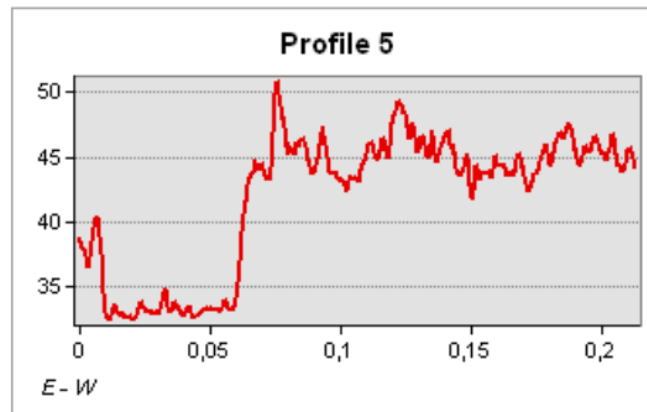
Imagen 63. Gráfica obtenida a partir del perfil de temperatura 5 de la imagen 62. Elaboración propia.
