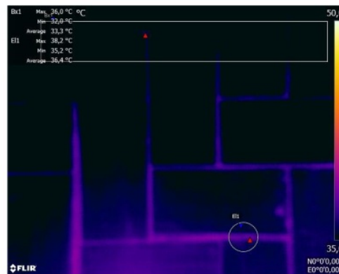
Imagen 48. Medición con ajuste de histograma de temperaturas entre 35-50°C, correspondiente al punto MC4-A, con señalización de valores de temperatura característicos de la imagen. Elaboración propia mediante el programa FLIRTools.
