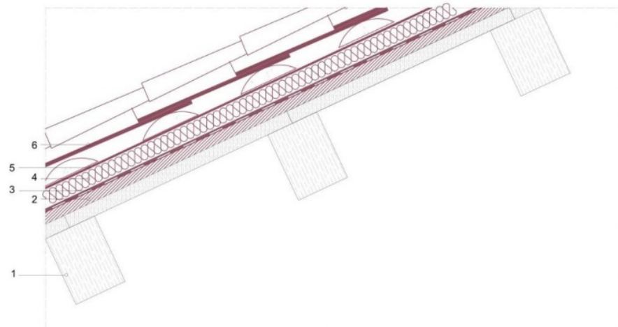
Detalle 2. Definición constructiva Cubierta 1. Elaboración propia
