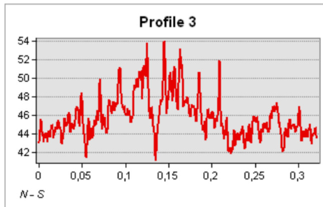
Imagen 65. Gráfica obtenida a partir del perfil de temperatura 3 de la imagen 64. Elaboración propia.
