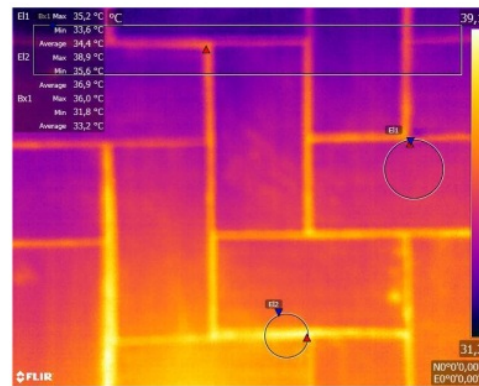
Imagen 47. Medición sin ajuste de histograma correspondiente al punto MC4-A, con señalización de valores de temperatura característicos de la imagen. Elaboración propia mediante el programa FLIRTools.
