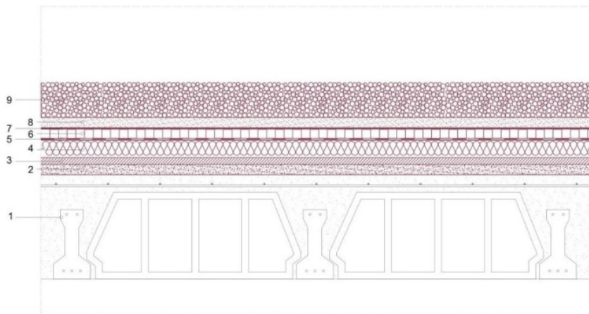
Detalle 4. Definición constructiva Cubierta 4. Elaboración propia
