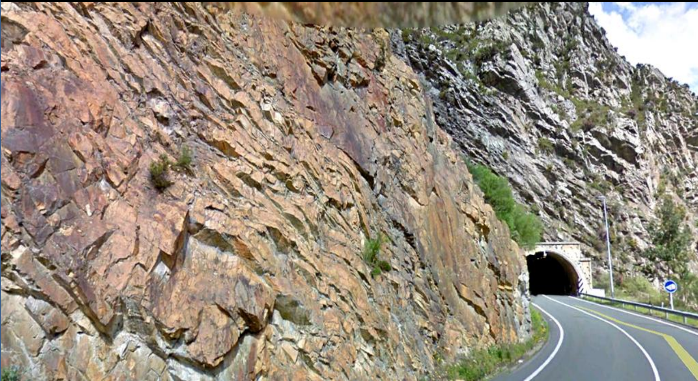
En las areniscas (Oville) Cambro-Ordovícico, en el Embalse de La Barca, Santa María, Tineo, Asturias. Centro N Hoja de Belmonte de Miranda
