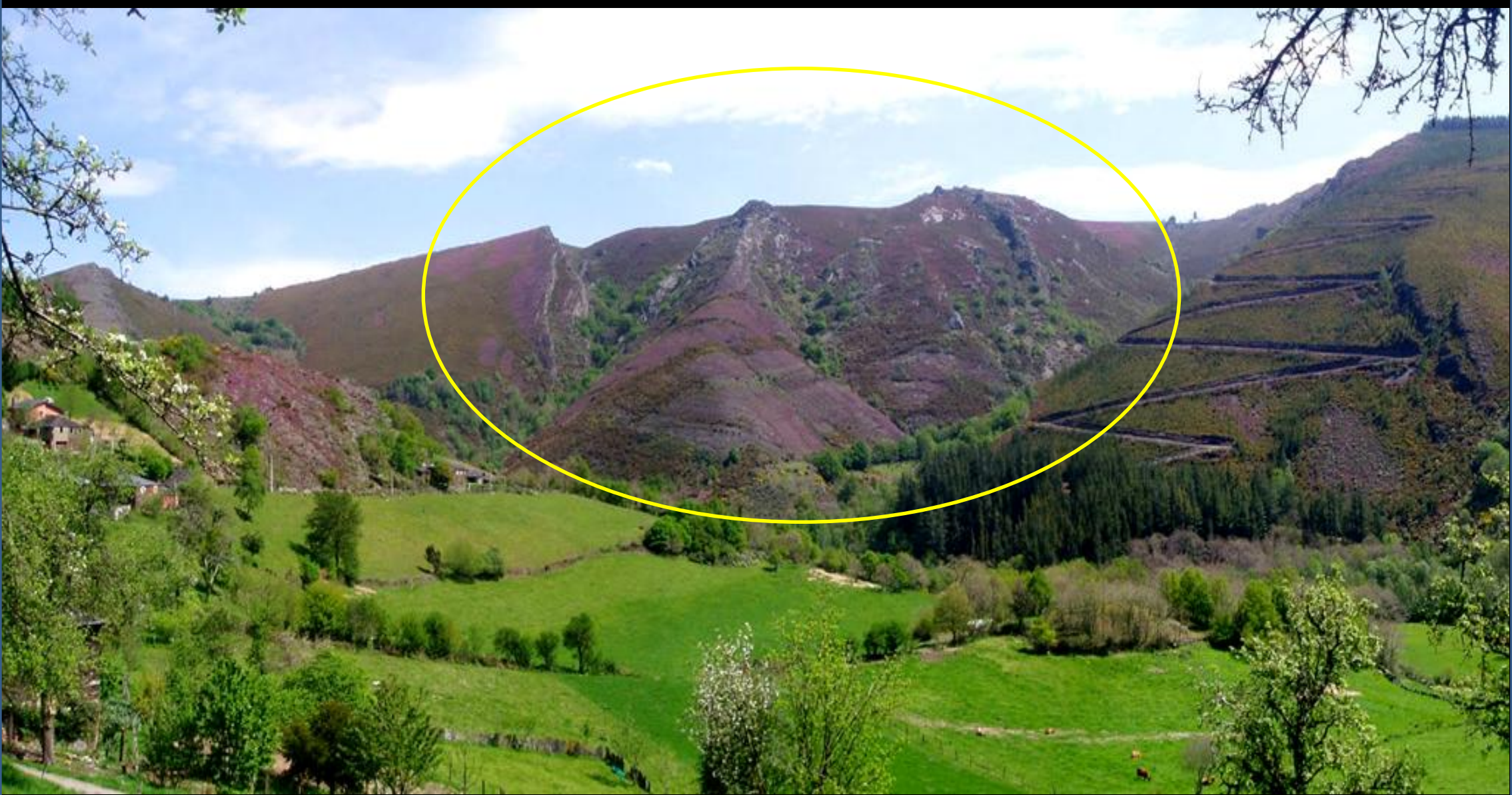
Tectónica en el Paleozoico. En Santa Eulalia de Oscos. Centro Hoja de San Martín de Oscos. Asturias. (por elcorty-Google)
