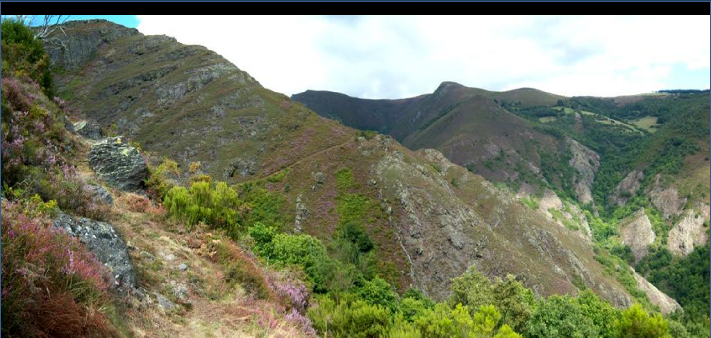
Pizarras negras (P. de Luarca) con metamorfismo, en NNE- NE Hoja- de San Martín de Oscos. Asturias. (por foristo-google)
