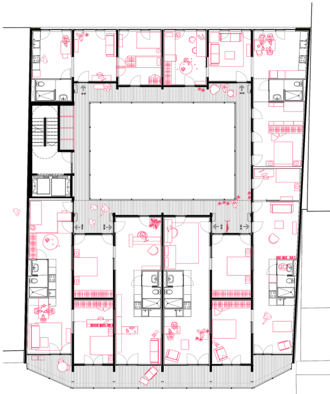
[F72]Planta tipo tercera i quarta Font: LaCol
