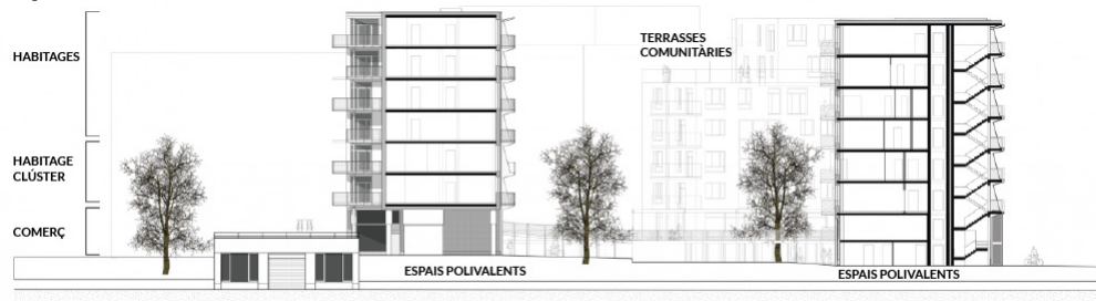
Querschnitt, Spreefeld Berlin © fatkoehl architekten
