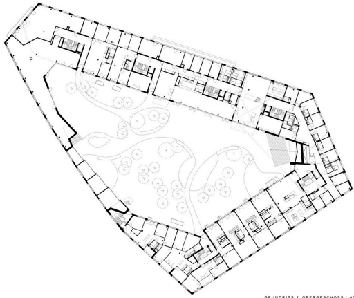
GRUNDRISS 2. OBERGESCHOSS 1:400
