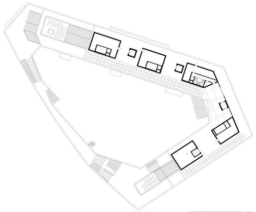
GRUNDRISS DACHGESCHOSS 1:400
