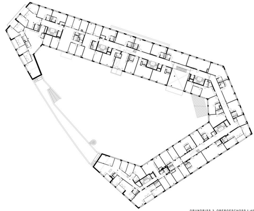
GRUNDRISS 3. OBERGESCHOSS 1:400
